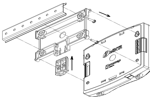
Рисунок 19. Вариант установки прибора через переходную планку на DIN-рейку(вид с задней крышки прибора)
