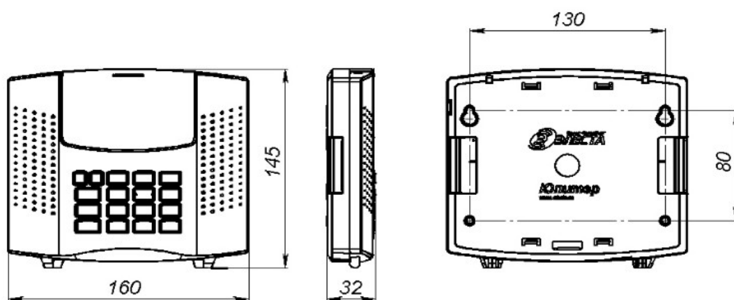
Рисунок 17. Габаритные и установочные размеры прибора
