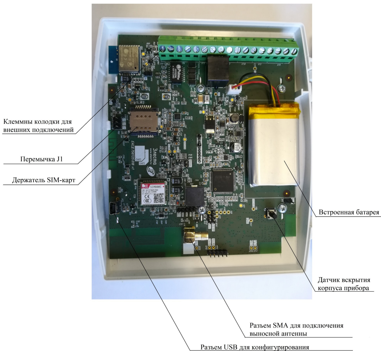
Рис. 5 Вид прибора с открытой крышкой
