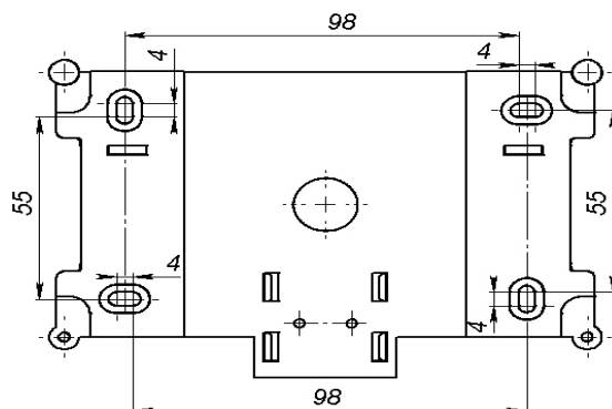
Рисунок 18. Габаритные размеры переходной планки
