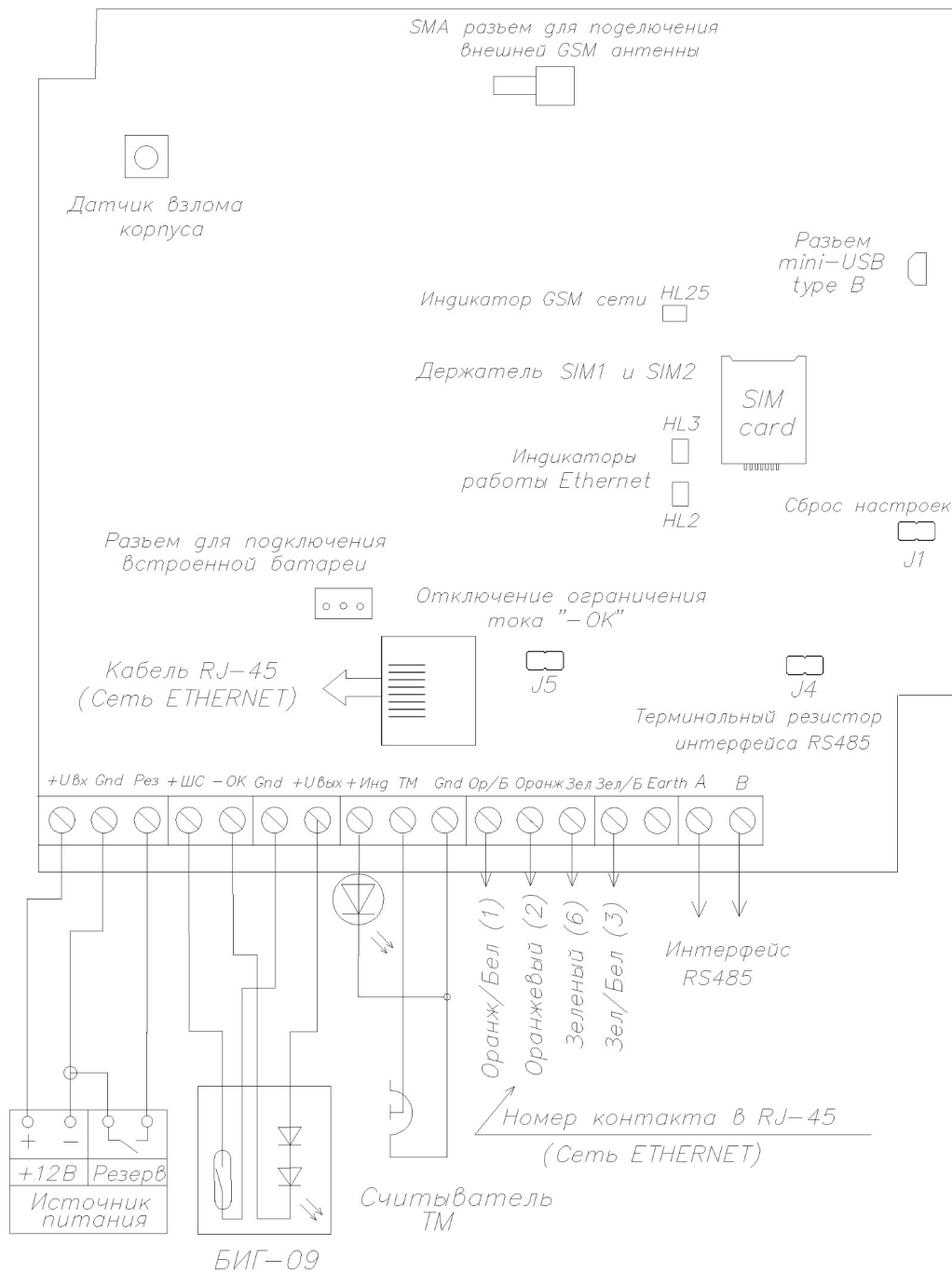
Рис. 10 Назначение разъемов прибора
