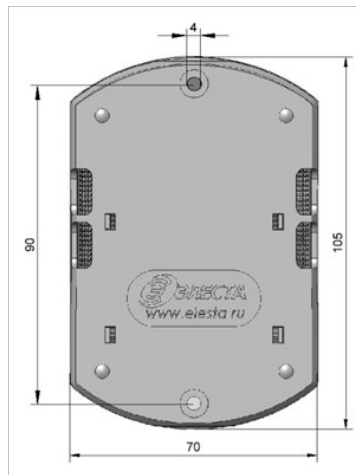
Рисунок 2 – Габаритные и установочные размеры прибора
