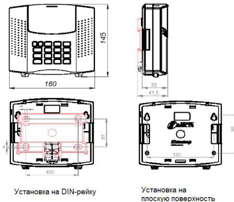
Рисунок 2. Габаритные и установочные размеры прибора
