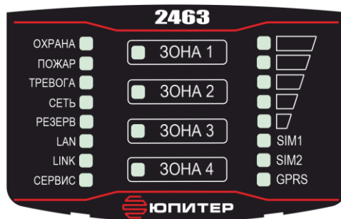
Рисунок 5 – Панель индикации УОО в исполнении Юпитер-2443, Юпитер-2445, Юпитер-2463 Подробное описание режимов работы индикаторов приведено в п.1.4.7.
