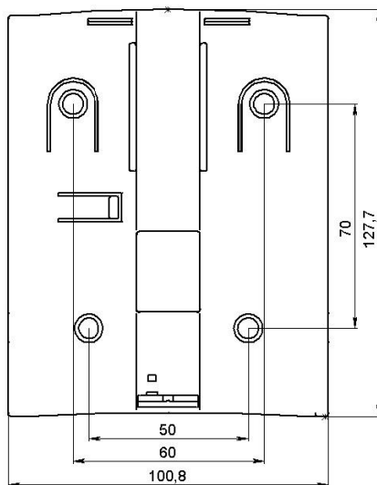
Рисунок 3 – Установочные размеры клавиатуры
