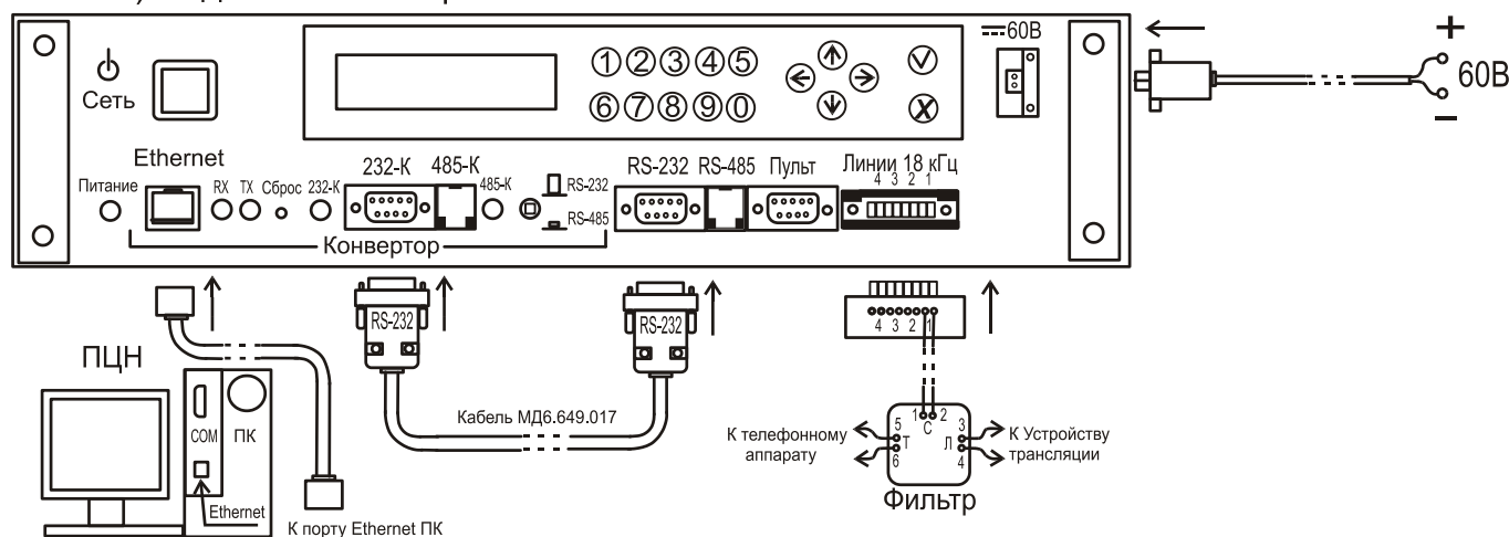
Рис.6.1 Подключение КПЦО-19
