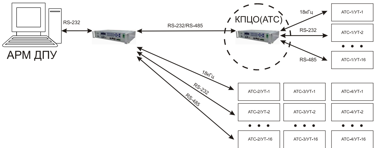
Рис. 7.1.2 Работа КПЦО-19 в режиме КПЦО-19 (АТЦ)
