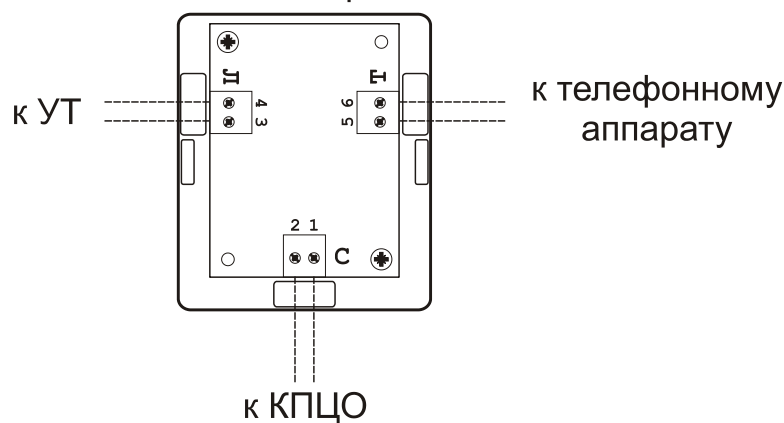
Рис.7.7.2.2 Включение фильтра 18кГц при использовании занятых телефонных линий.
