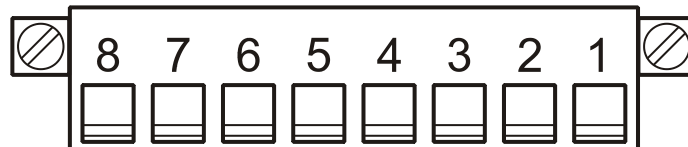
Рис.7.7.2.1 Назначение контактов разъема каналов «18кГц».
