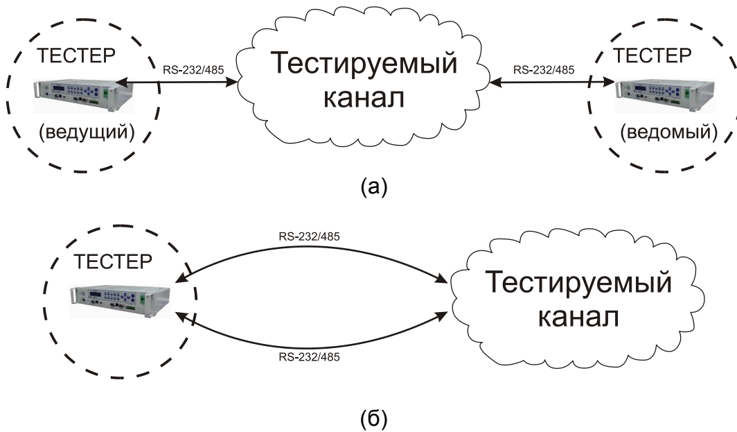
Рис. 7.1.3 Работа КПЦО-19 в режиме ТЕСТЕР: а) тестирование обычного канала, б) тестирование закольцованного канала.
