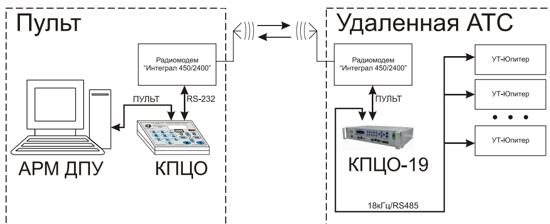
Рис. 7.5.3.3 Цифровой канал на основе радиомодемов.
