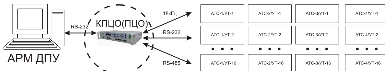
Рис. 7.1.1а Работа КПЦО-19 в режиме КПЦО(ПЦО), прямое подключение.
