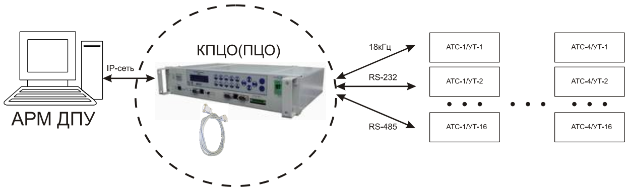
Рис. 7.1.16 Работа КПЦО-19 в режиме КПЦО(ПКЦО), подключение по IP-сети.
