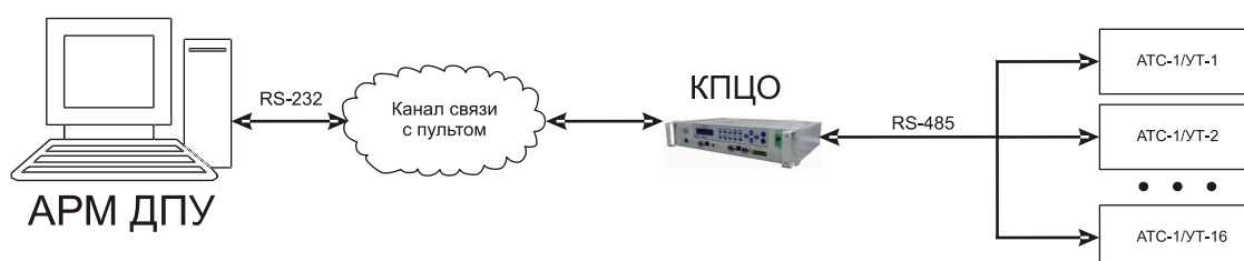
Рис. 7.3.2.2 КПЦО-19, непосредственно контролирующей УТ по каналу RS-485.
