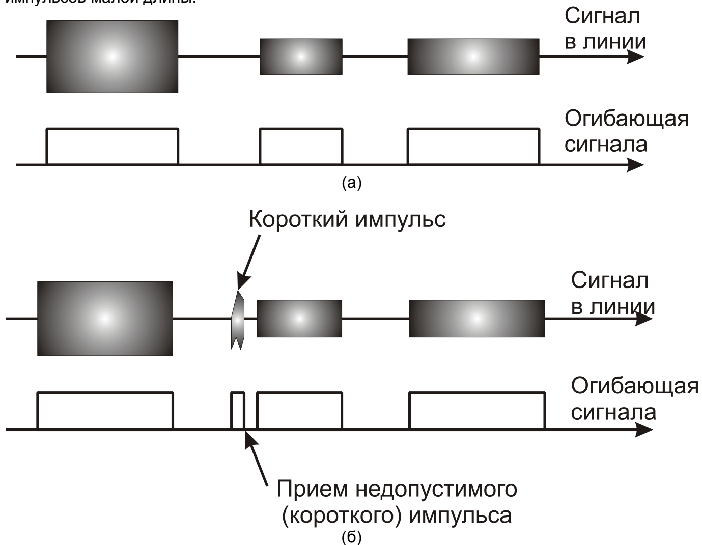
Рис. 7.3.6.2. Результат приема импульсов от УТ: а) помех нет, б) на линии помехи
