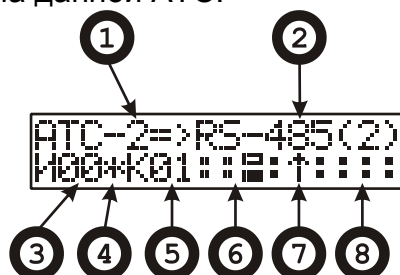
Рис.7.2.7-10. Рабочий экран АТС.
