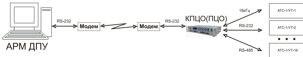
Рис. 7.5.3.2 Цифровой канал на основе модемов.
