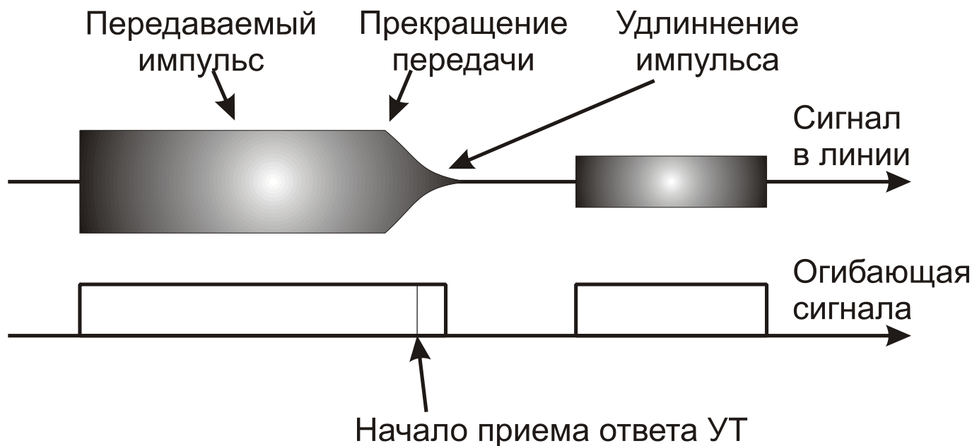
Рис. 7.3.6.3. Удлинение остаточного сигнала, после окончания передачи
