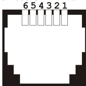
Рис.7.7.7 Назначение контактов разъема канала «RS-485».
