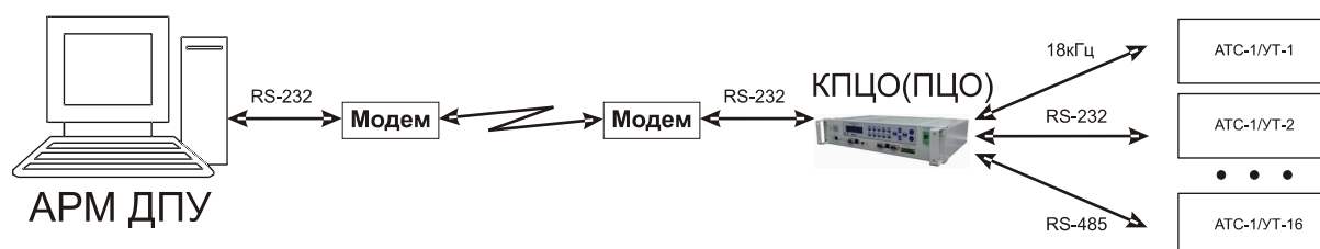
Рис. 7.3.2.1 Включение «удаленного» КПЦО-19 по модемному каналу.
