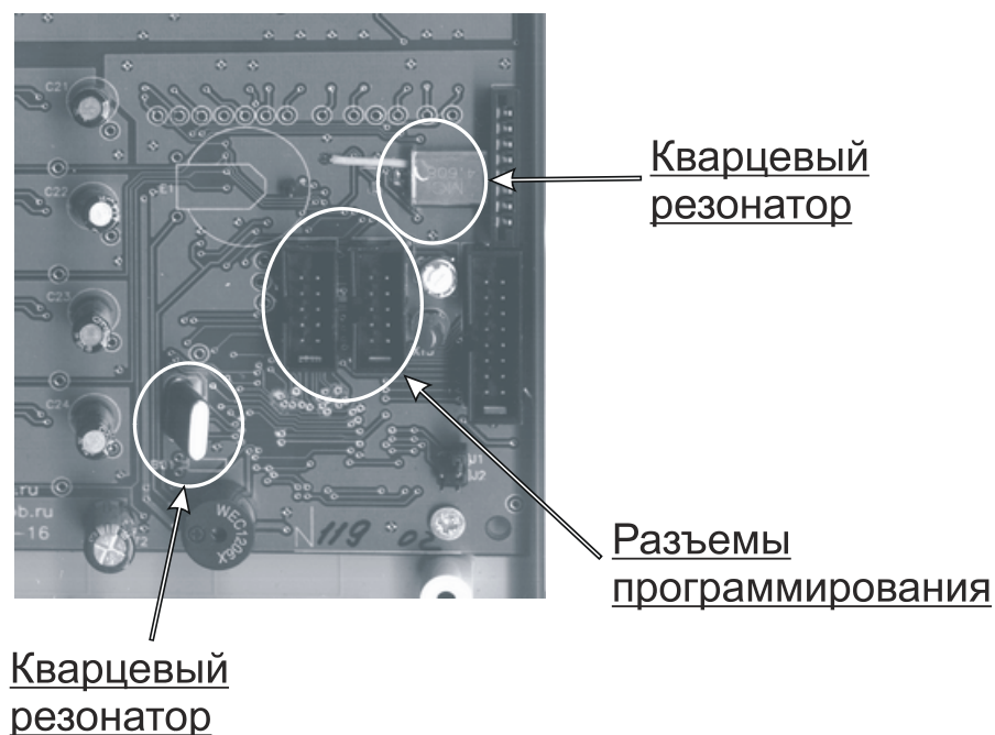
Рис.7.6.3. Размещение кварцевого резонатора для Atmega128 (два резонатора)
