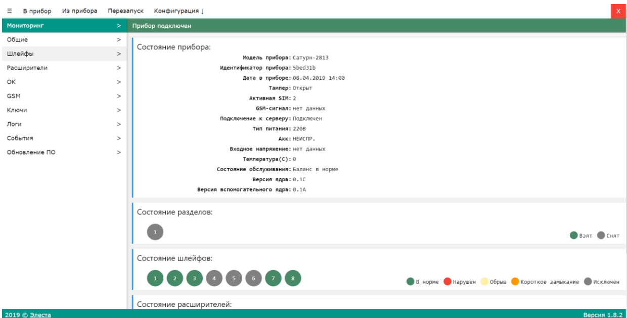
Рисунок 15: Удаленный конфигуратор прибора в Шлюз КРОС
