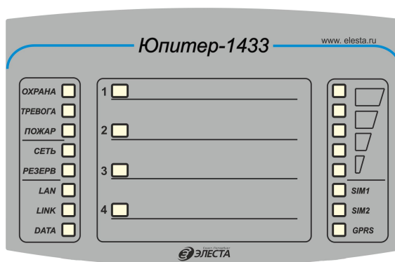
Рисунок 3. Внешний вид панели индикации Юпитер-1433
