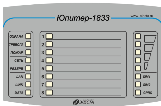
Рисунок 4. Внешний вид панели индикации Юпитер-1833
