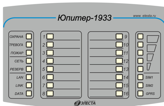
Рисунок 5. Внешний вид панели индикации Юпитер-1933
