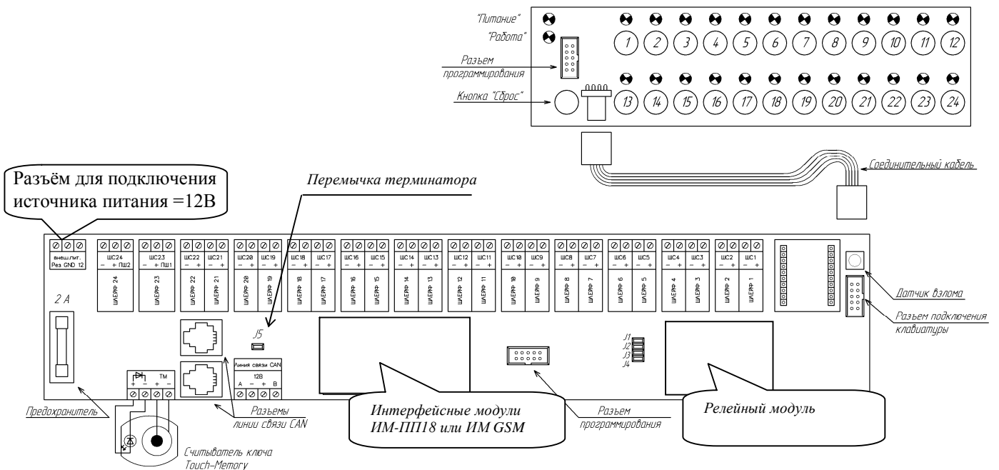
Рис. 5 Подключение ППКОП24к
