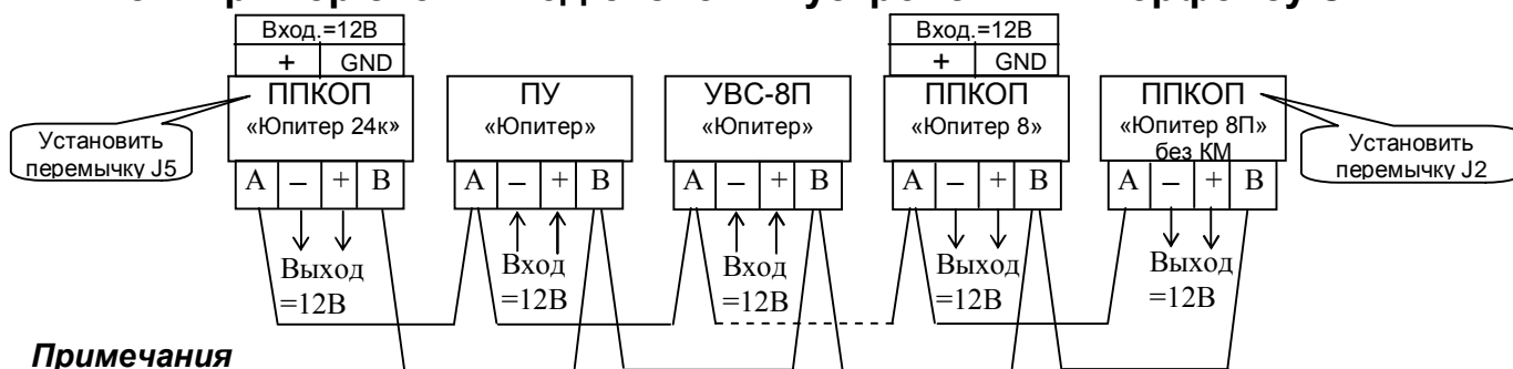
Рис.1 Пример схемы подключения устройств к интерфейсу CAN
