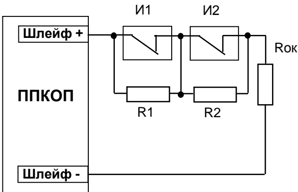
Рис.3 Примеры шлейфов охранной сигнализации
