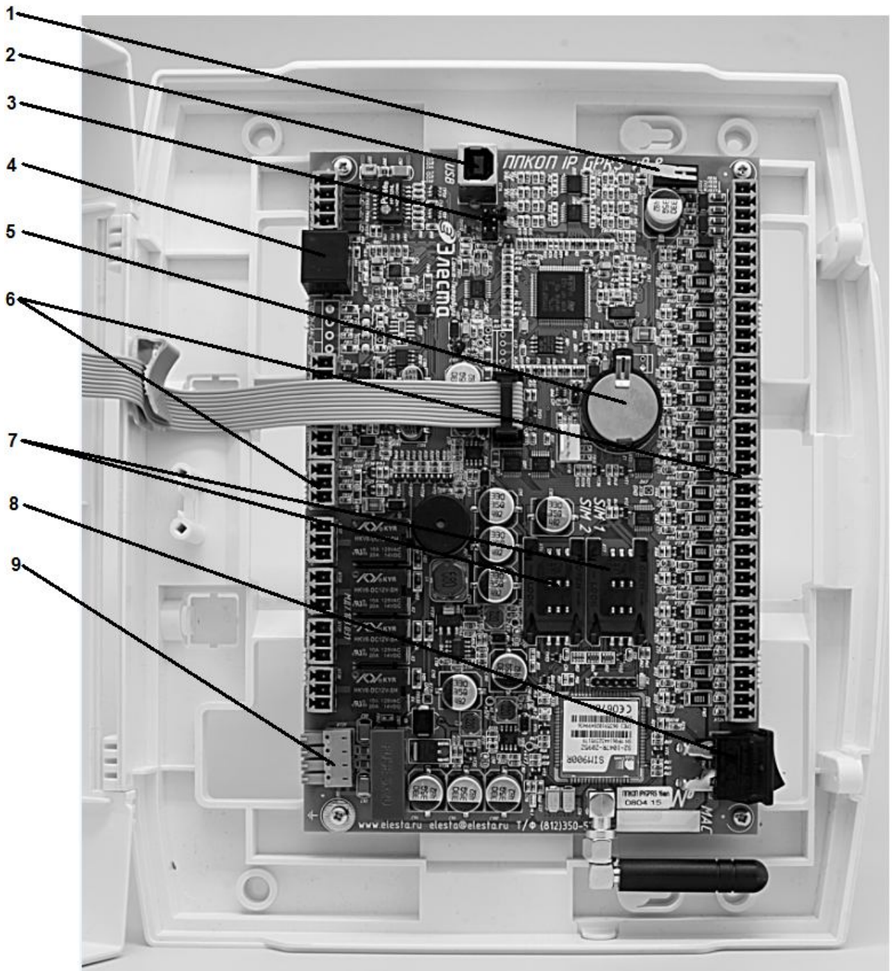
Рисунок 2.4. Вид прибора с открытой крышкой
