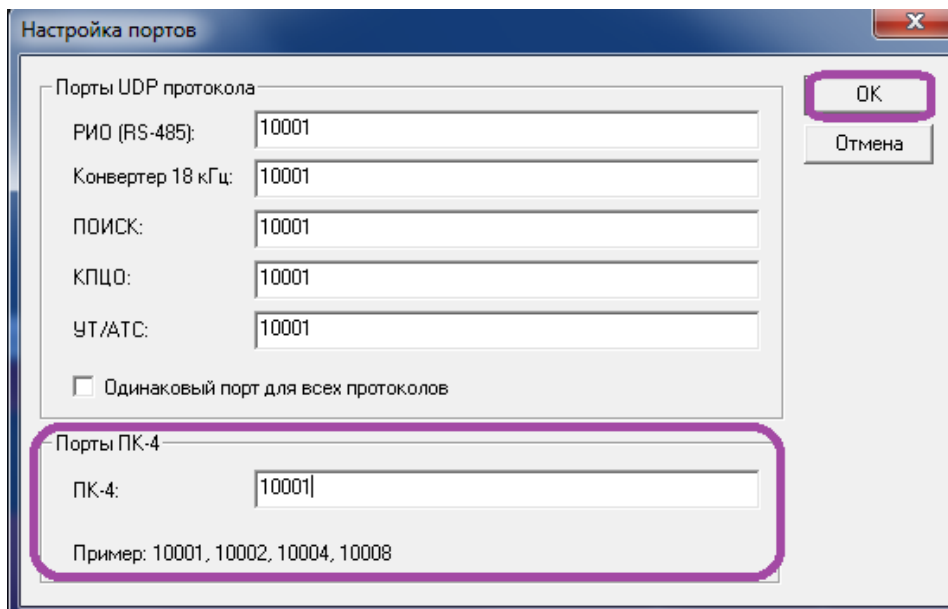
Рисунок 31: «Настройка портов»
