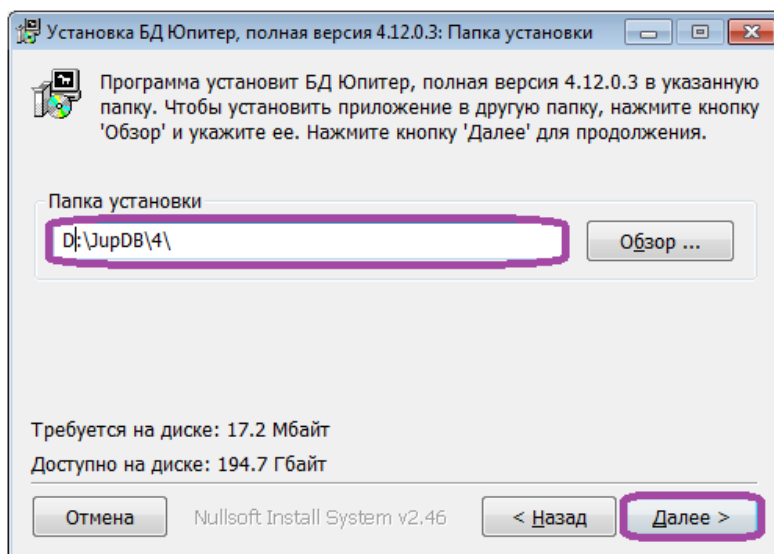
Рисунок 9: Папка установки
