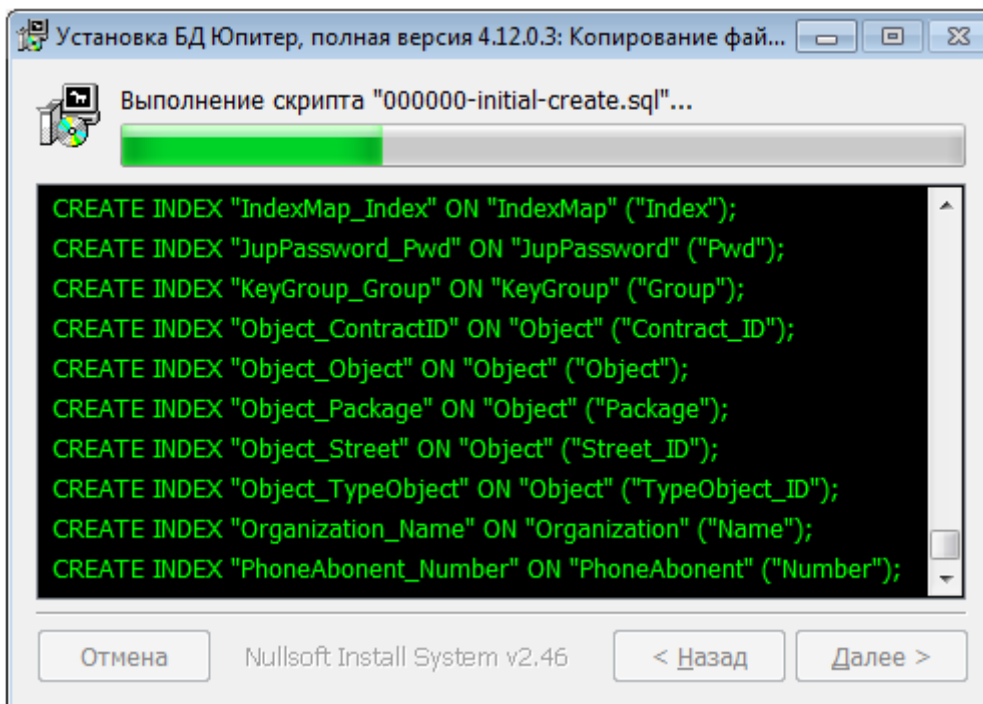
Рисунок 13: Процесс установки
