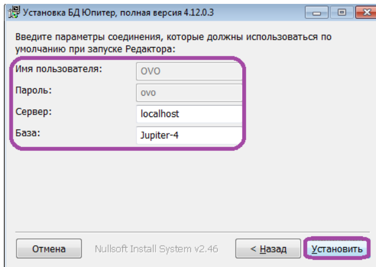
Рисунок 12: Параметры соединения
