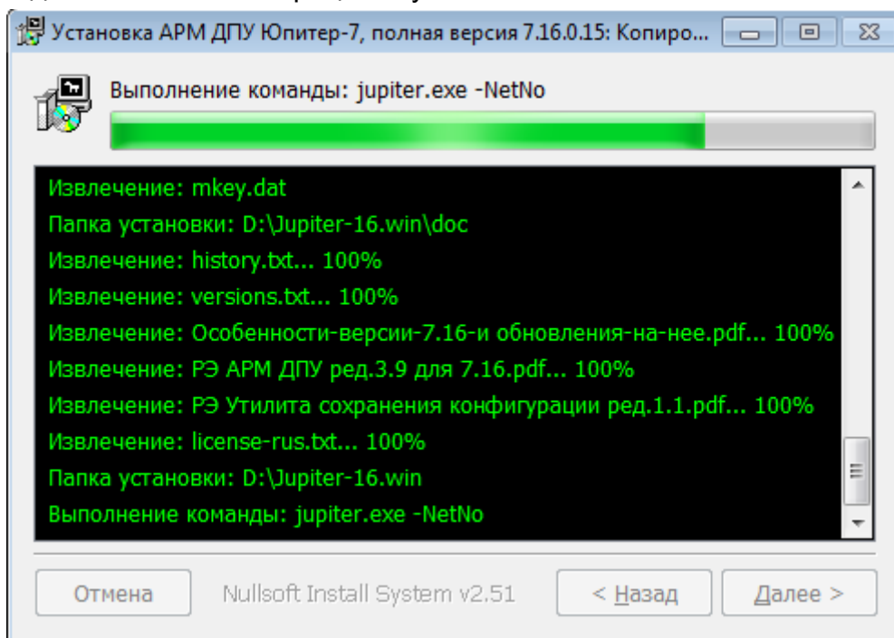
Рисунок 23: Процесс установки.
