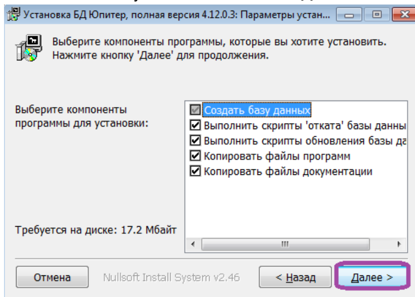
Рисунок 8: Компоненты установки
