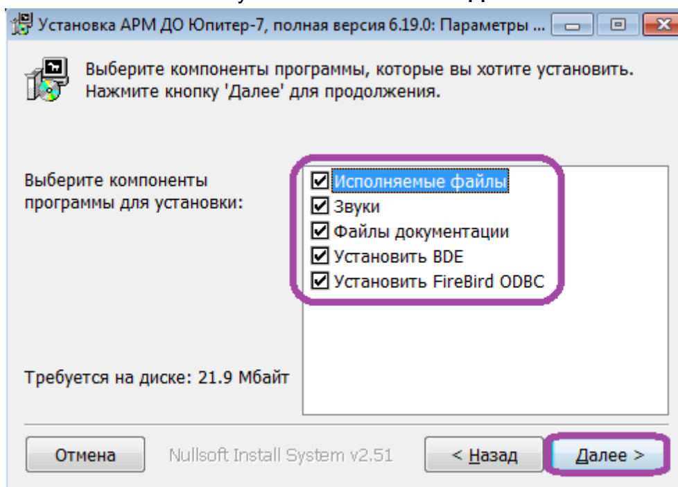
Рисунок 33: Компоненты установки.
