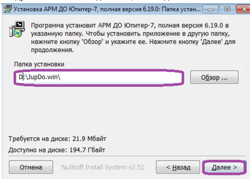
Рисунок 34: Папка установки.
