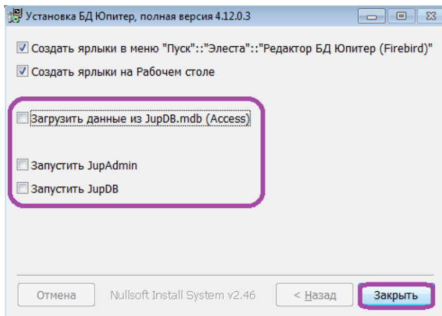
Рисунок 15: Завершение установки
