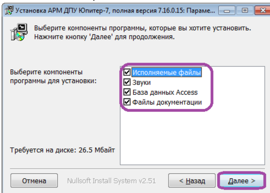
Рисунок 20: Компоненты установки.
