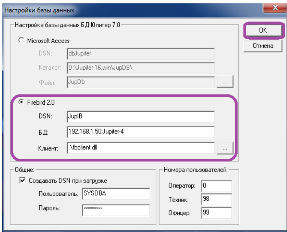
Рисунок 48: Подключение базы данных к клиенту
