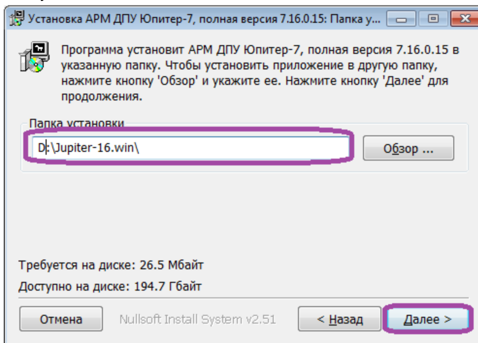
Рисунок 40: Папка установки
