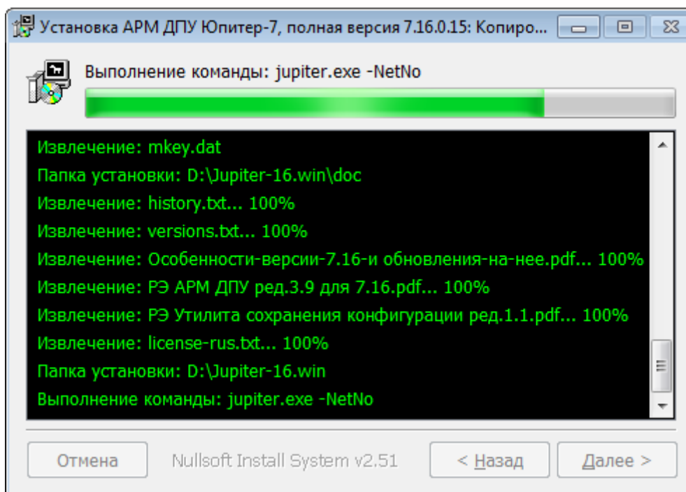
Рисунок 23: Процесс установки.
