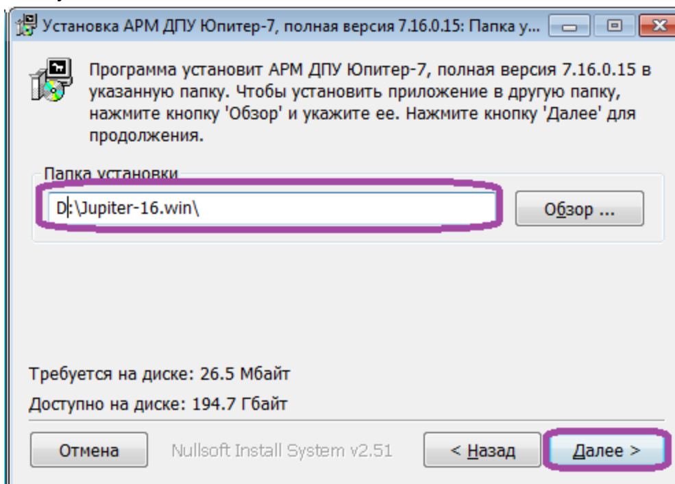
Рисунок 21: Папка установки.
