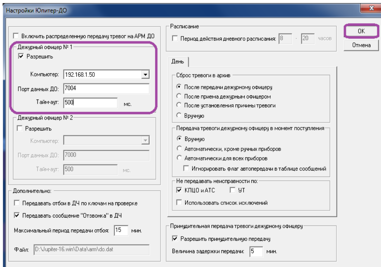
Рисунок 85: Окно «Настройки Юпитер-ДО»
