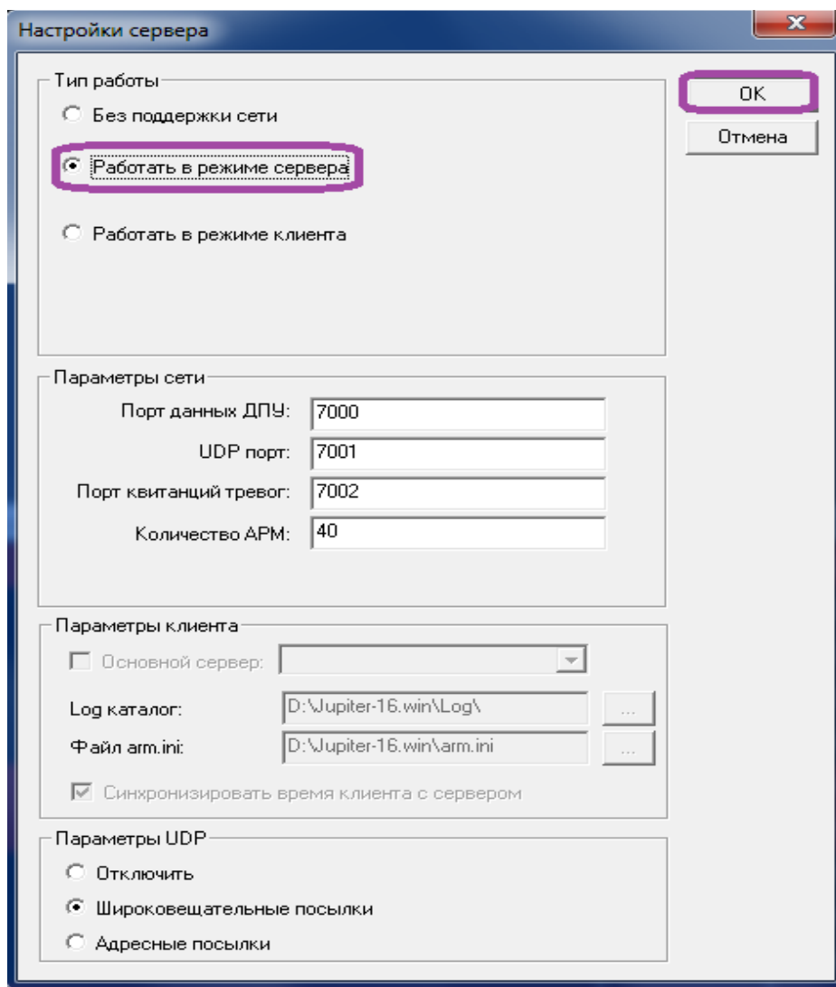
Рисунок 29: Перевод АРМ ДПУ «Юпитер» в режим сервера
