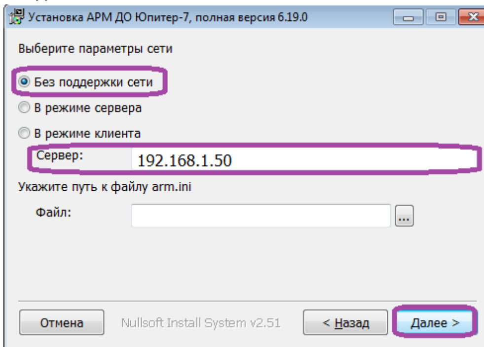
Рисунок 60: Выбор режима установки
