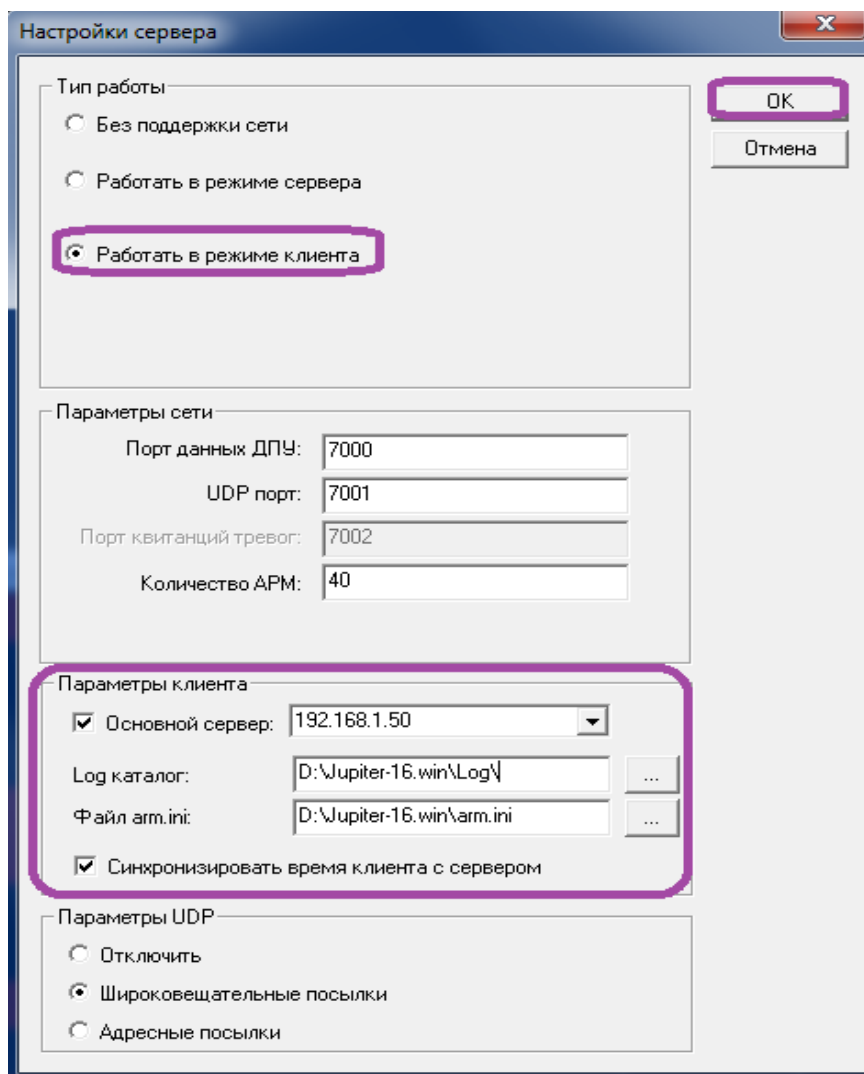
Рисунок 54: Окно « Настройки сервера » в режиме клиента.
