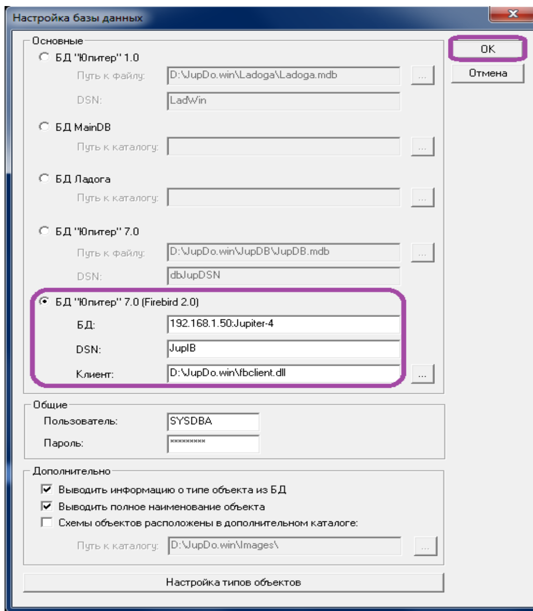
Рисунок 80: Подключение базы данных
