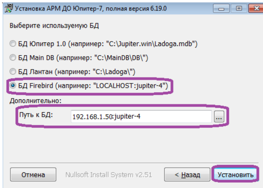
Рисунок 62: Выбор используемой БД
