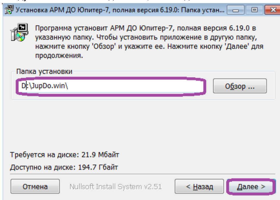
Рисунок 58: Папка установки.
