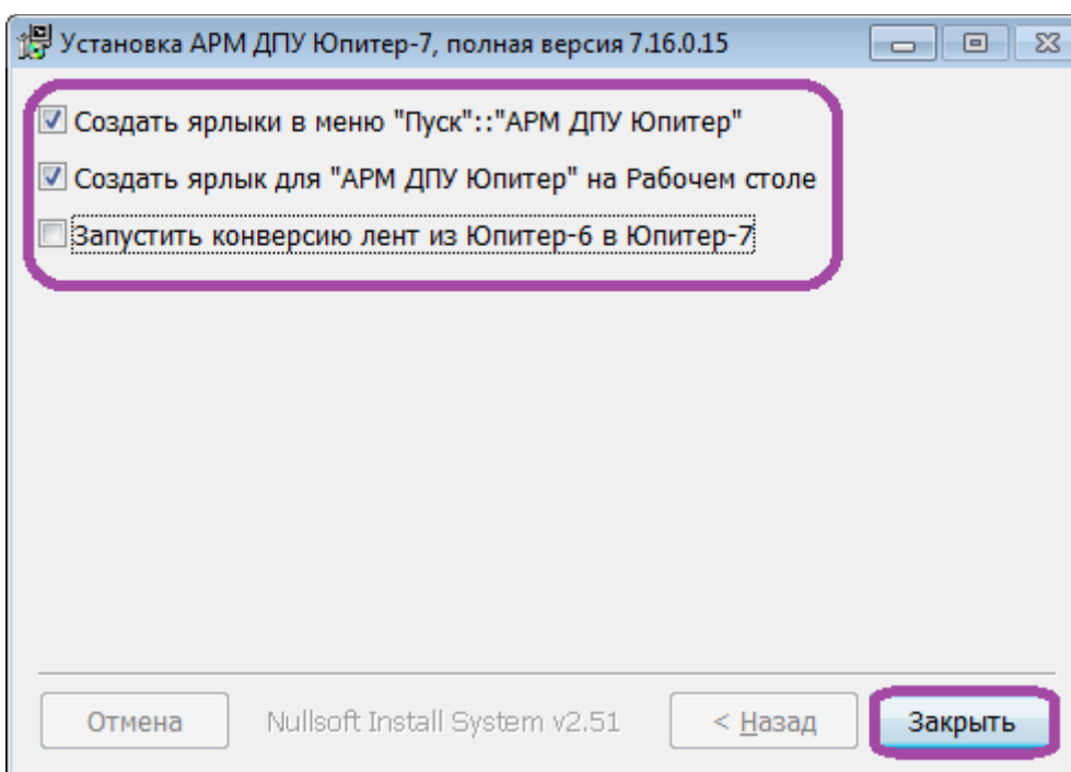
Рисунок 45: Завершение установки.
