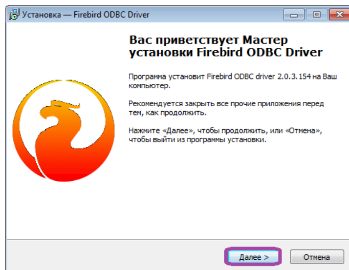
Рисунок 69: Начало установки
