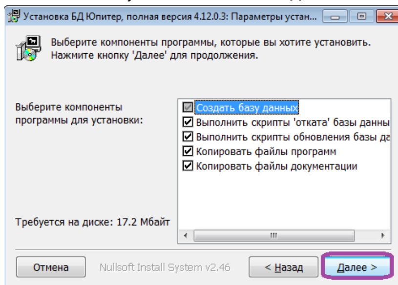
Рисунок 9: Компоненты установки
