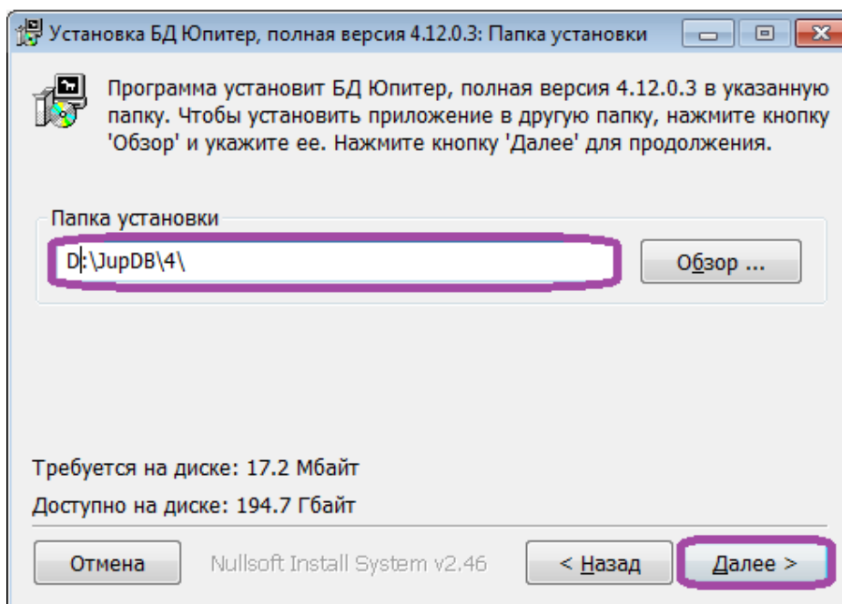
Рисунок 10: Папка установки
