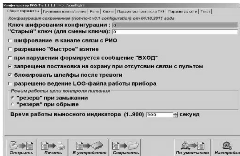
Рис.5 Главное окно программы.
