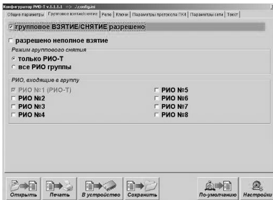
Рис.6 Закладка Групповое взятие/снятие.
