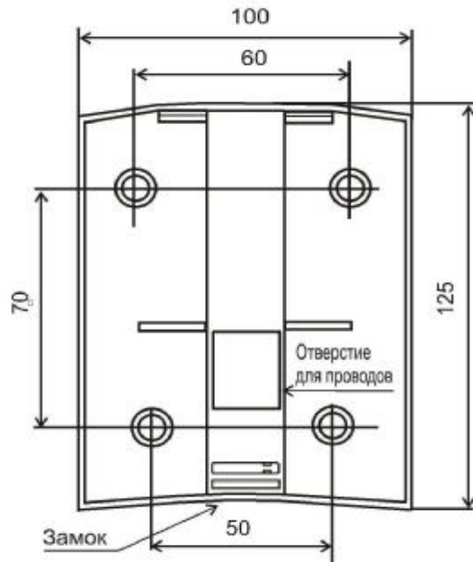
Рис.2 Установочные размеры РИО-Т
