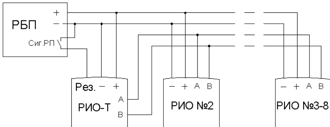
а) Схема с одним РБП:
