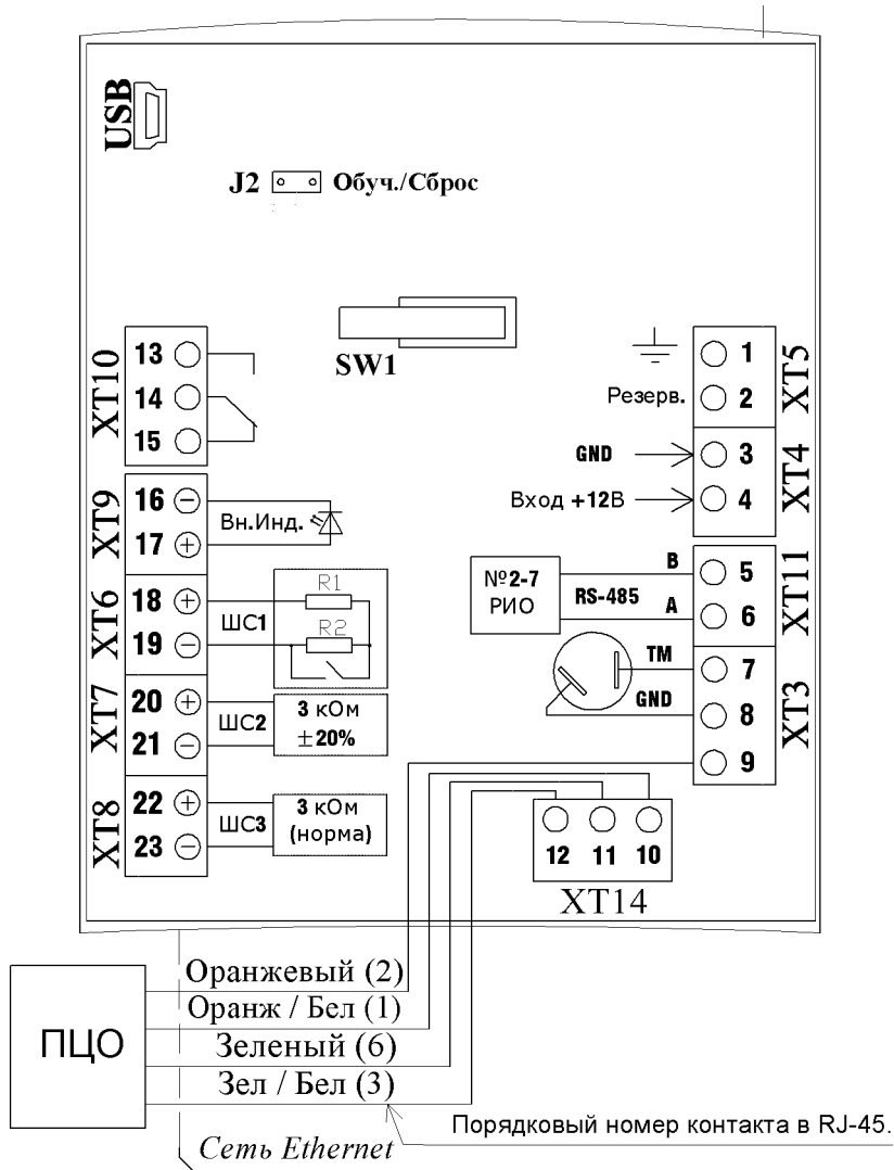
Рис.1 Внешний вид РИО-Т
