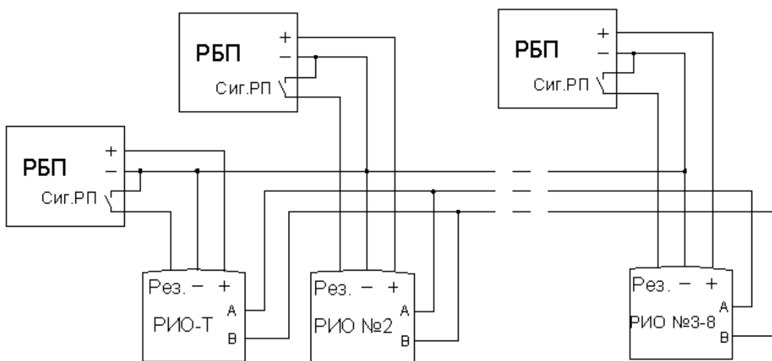
б) Схема с РБП для каждого RIO
