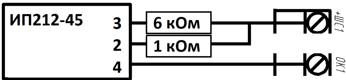
Рисунок 3.2. Схема подключения пожарного извещателя через ОК.
