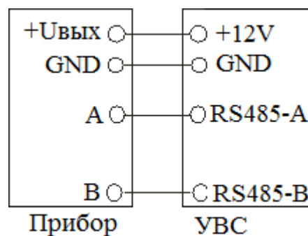
Рисунок 3.5. Подключение УВС по RS485
