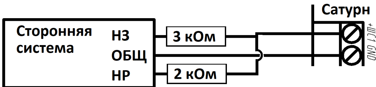
Рисунок 3.1. Схема подключения сторонней системы с релейным выходом.
