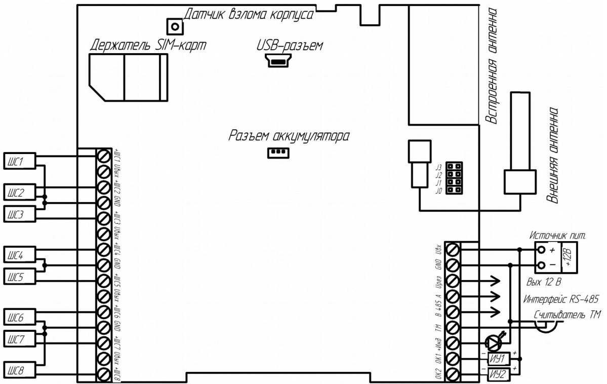
Рисунок 2.9. Назначение разъемов УОО «Сатурн-2813» и УОО «Сатурн-2814»
