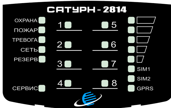
Рисунок 2.7. Панель индикации УОО в исполнении Сатурн-2814
