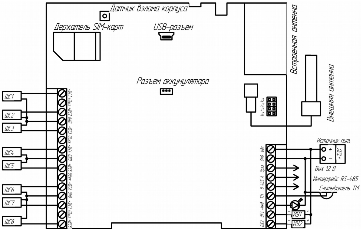
Рисунок 2.9. Назначение разъемов УОО «Сатурн-2813» и УОО «Сатурн-2814»
