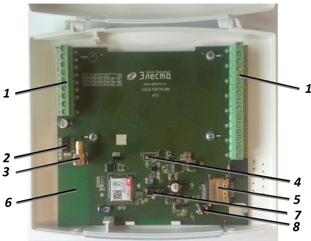
Рисунок 2.4. Сатурн-2813/Сатурн-2814 с открытой крышкой
