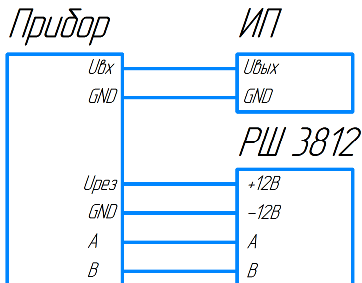
Рисунок 3.1. Подключение питания
