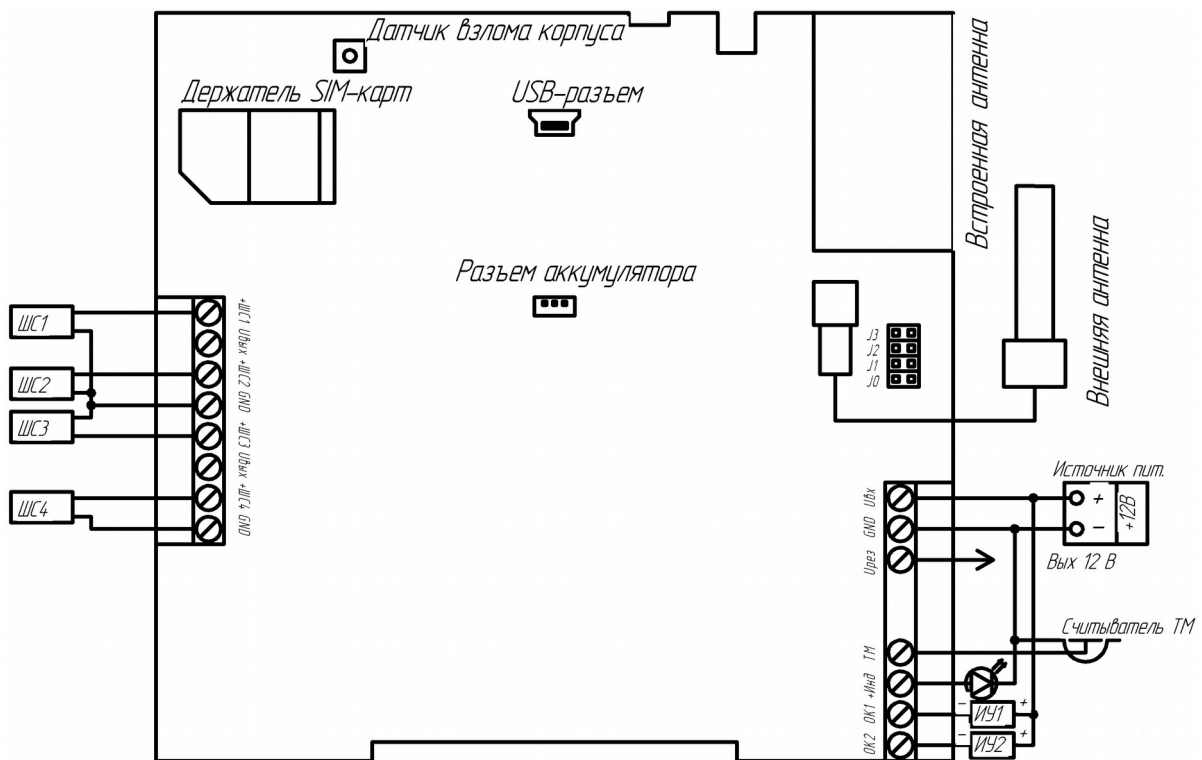
Рисунок 2.8. Назначение разъемов УОО «Сатурн-2413»
