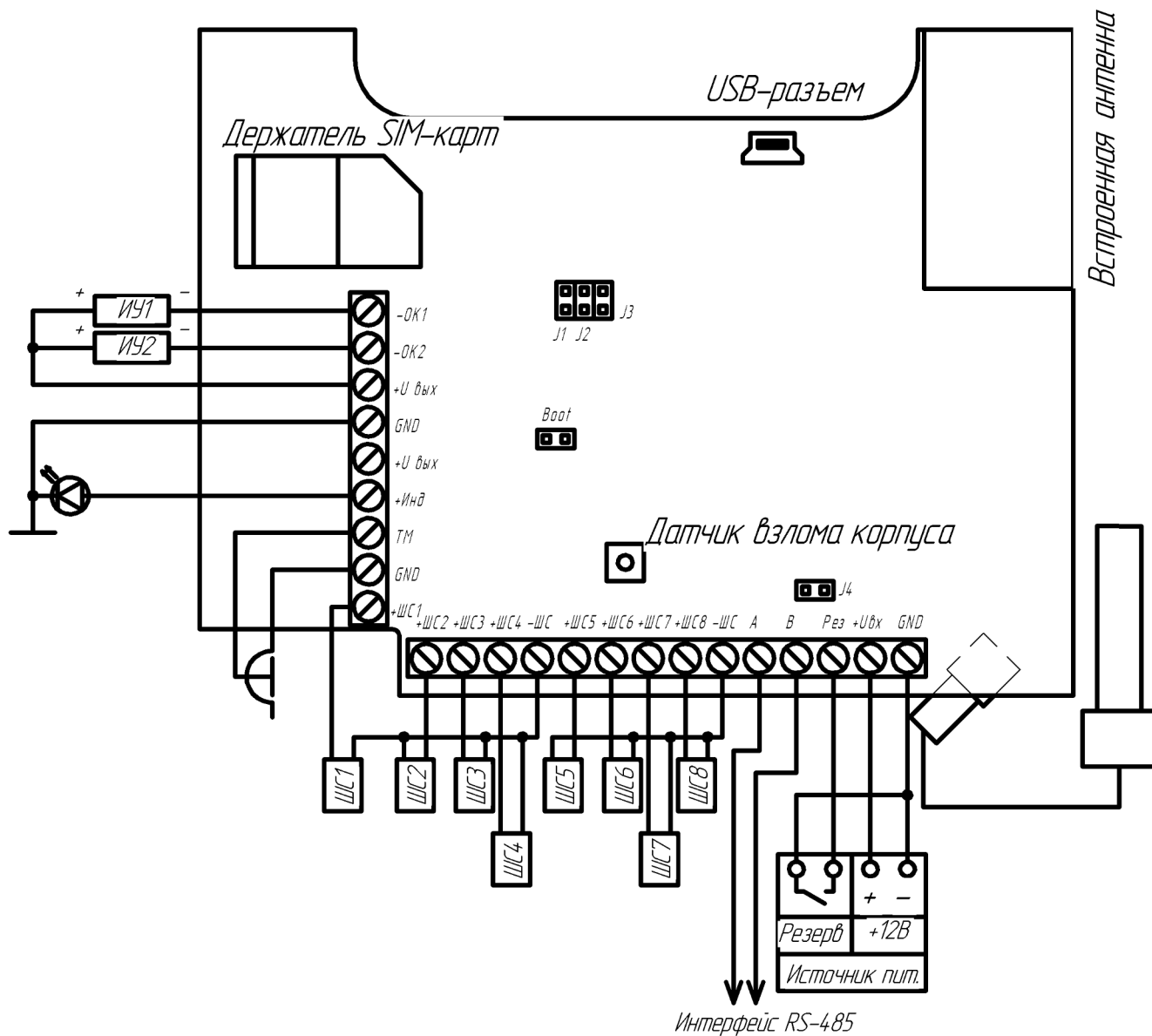
Рисунок 2.2. Назначение разъемов прибора
