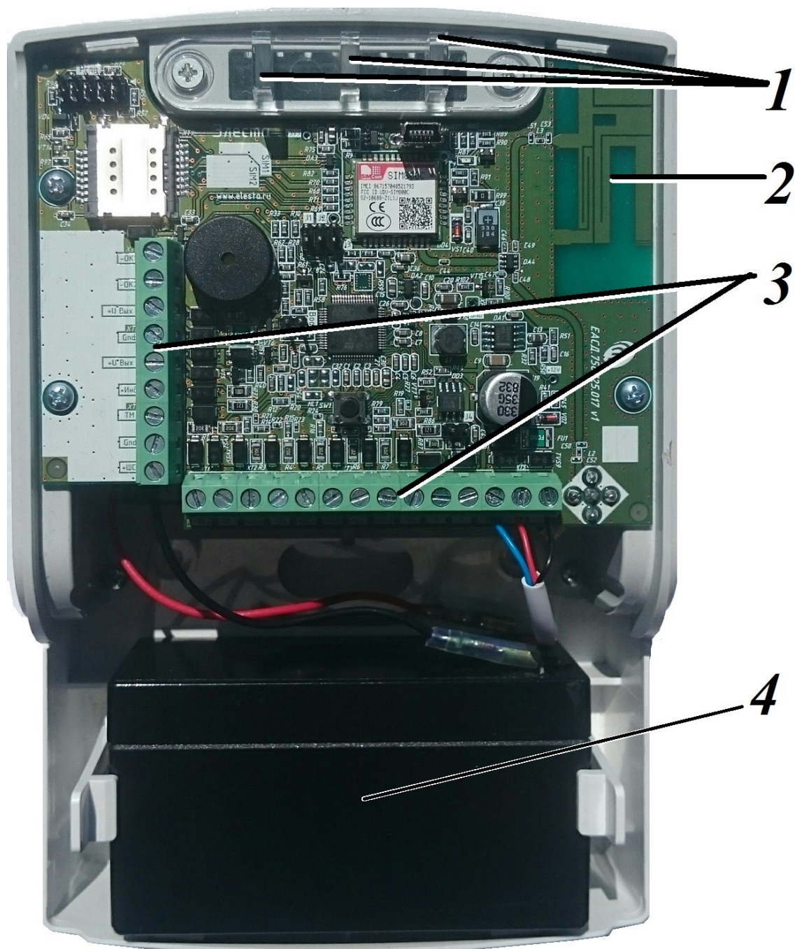
Рисунок 2.1. Прибор Сатурн-2818 с открытой крышкой
