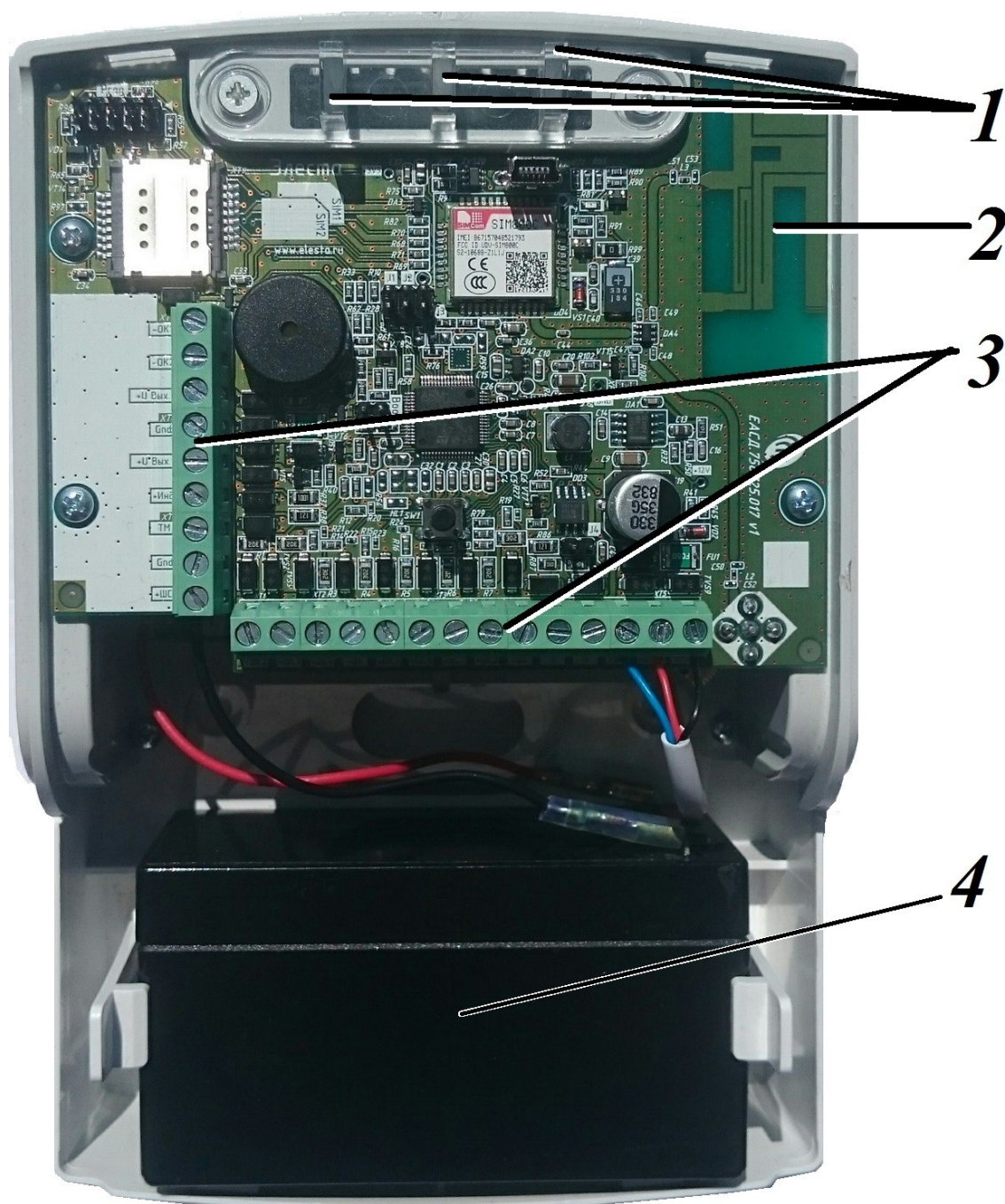
Рисунок 2.1. Прибор Сатурн-2818 с открытой крышкой
