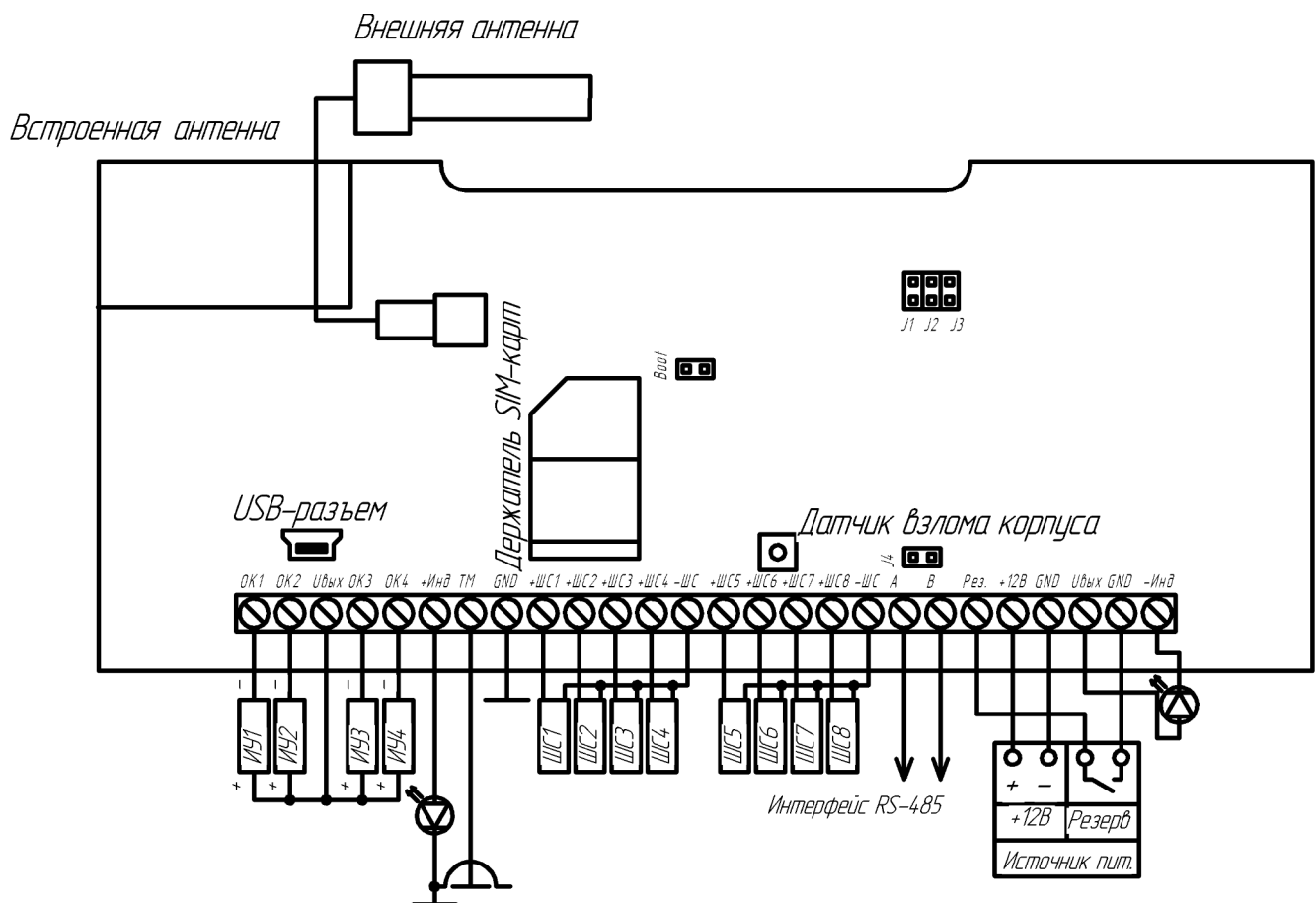
Рисунок 2.2. Назначение разъемов прибора
