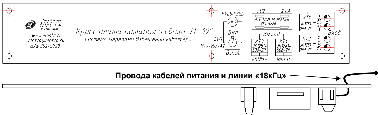
Рис.4. Кросс плата питания и связи УТ-19”
