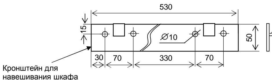
Рис.1. Размеры для установки кронштейна для навешивания шкафа на стену
