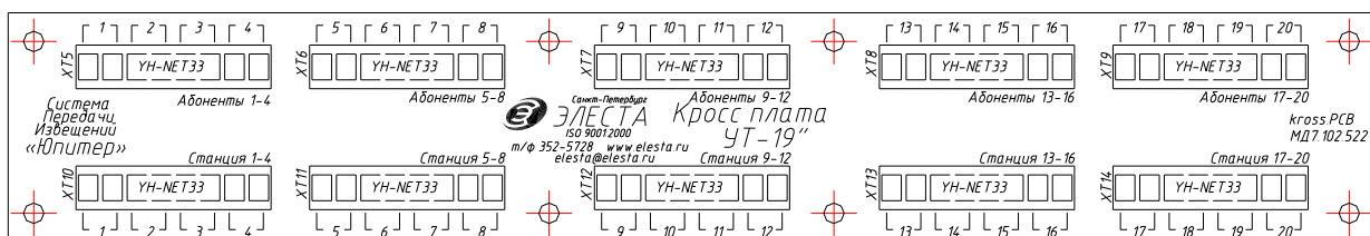
Рис.5. Кросс плата УТ-19” (Вид со стороны колодок для внешних подключений)
