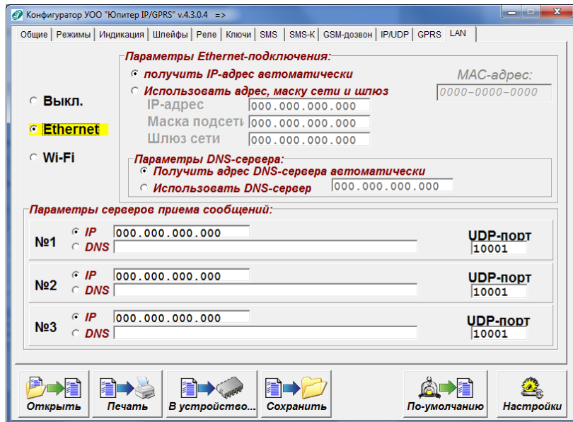
Рисунок 15. Окно программы Конфигуратора, вкладка «LAN» с установленным переключателем «Ethernet»
