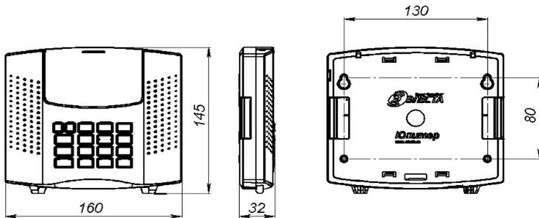
Рисунок 17. Габаритные и установочные размеры прибора
