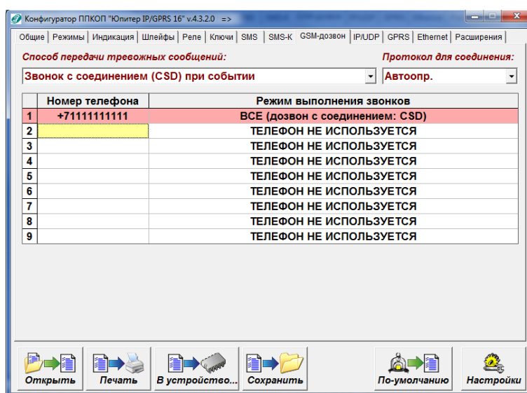
Рисунок 9. Окно программы Конфигуратора, вкладка «GSM-дозвон». Настройка дозвона с соединением (CSD)
