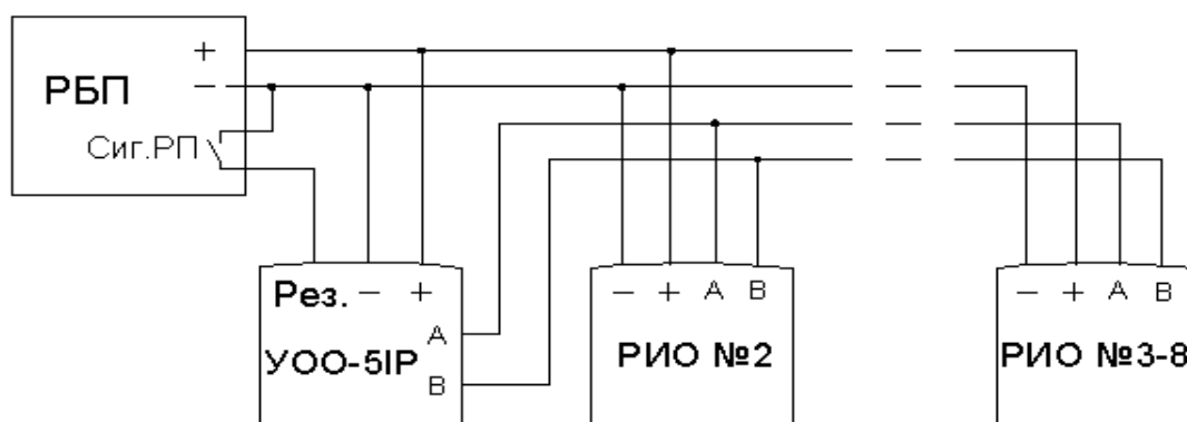
а) Схема с одним РБП
