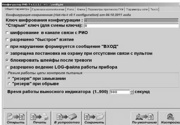
Рис.5 Главное окно программы.
