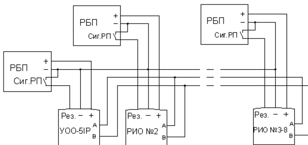
б) Схема с РБП для каждого РИО
