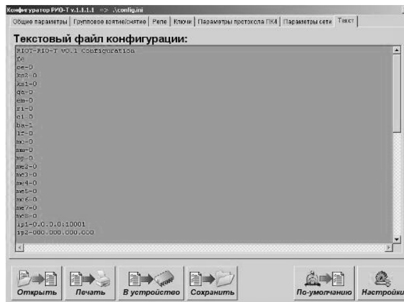
Рис.11 Закладка Текст
