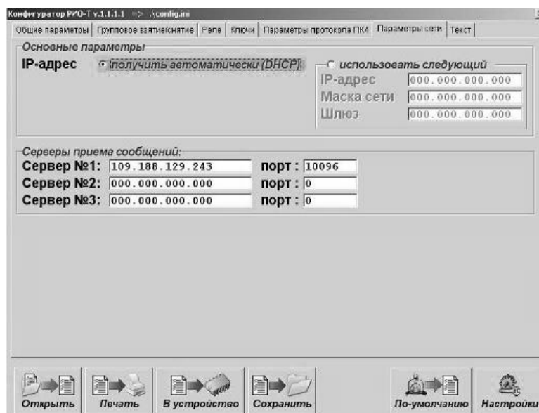
Рис.10 Параметры сети
