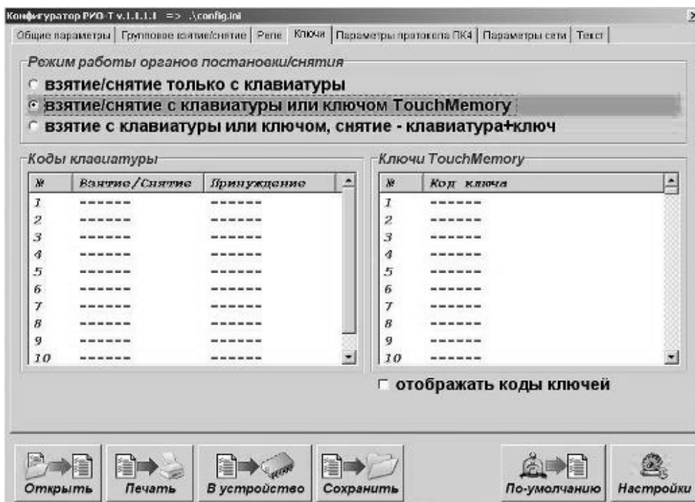
Рис.8 Закладка реле
