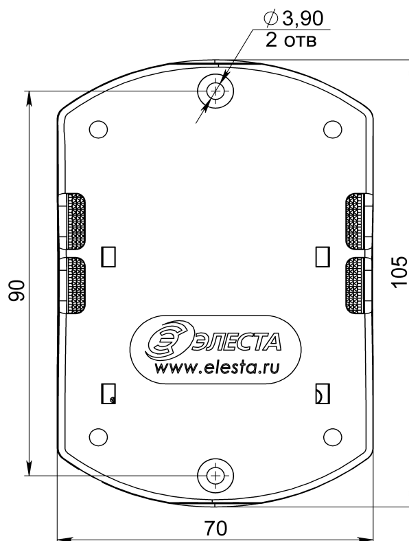
Рисунок 6. Габаритные и установочные размеры прибора Юпитер-2021
