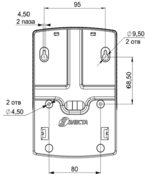
Рисунок 7. Габаритные и установочные размеры прибора Юпитер -2028
