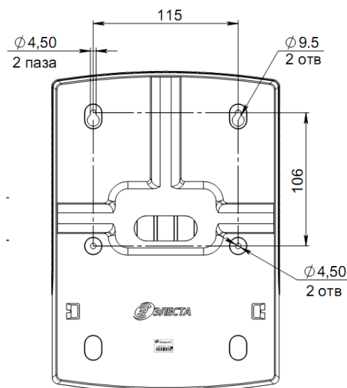
Рисунок 8. Габаритные и установочные размеры прибора Юпитер -2029
