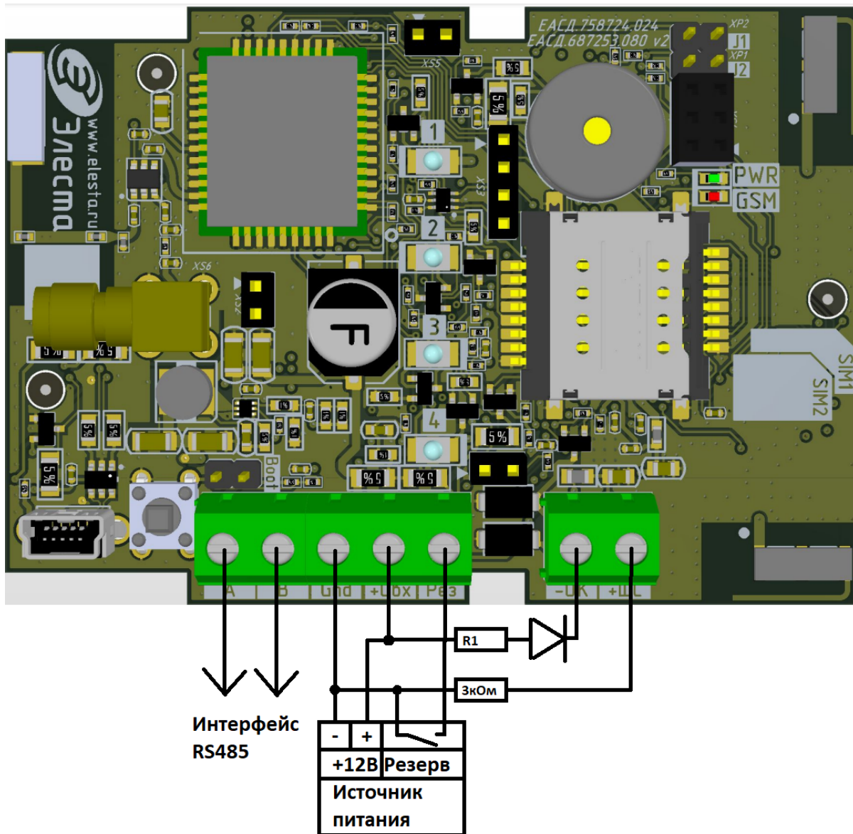
Рис. 5 Назначение разъемов прибора
