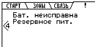
Рис. 3.6 Экран тревожных сообщений и неисправности «!».
