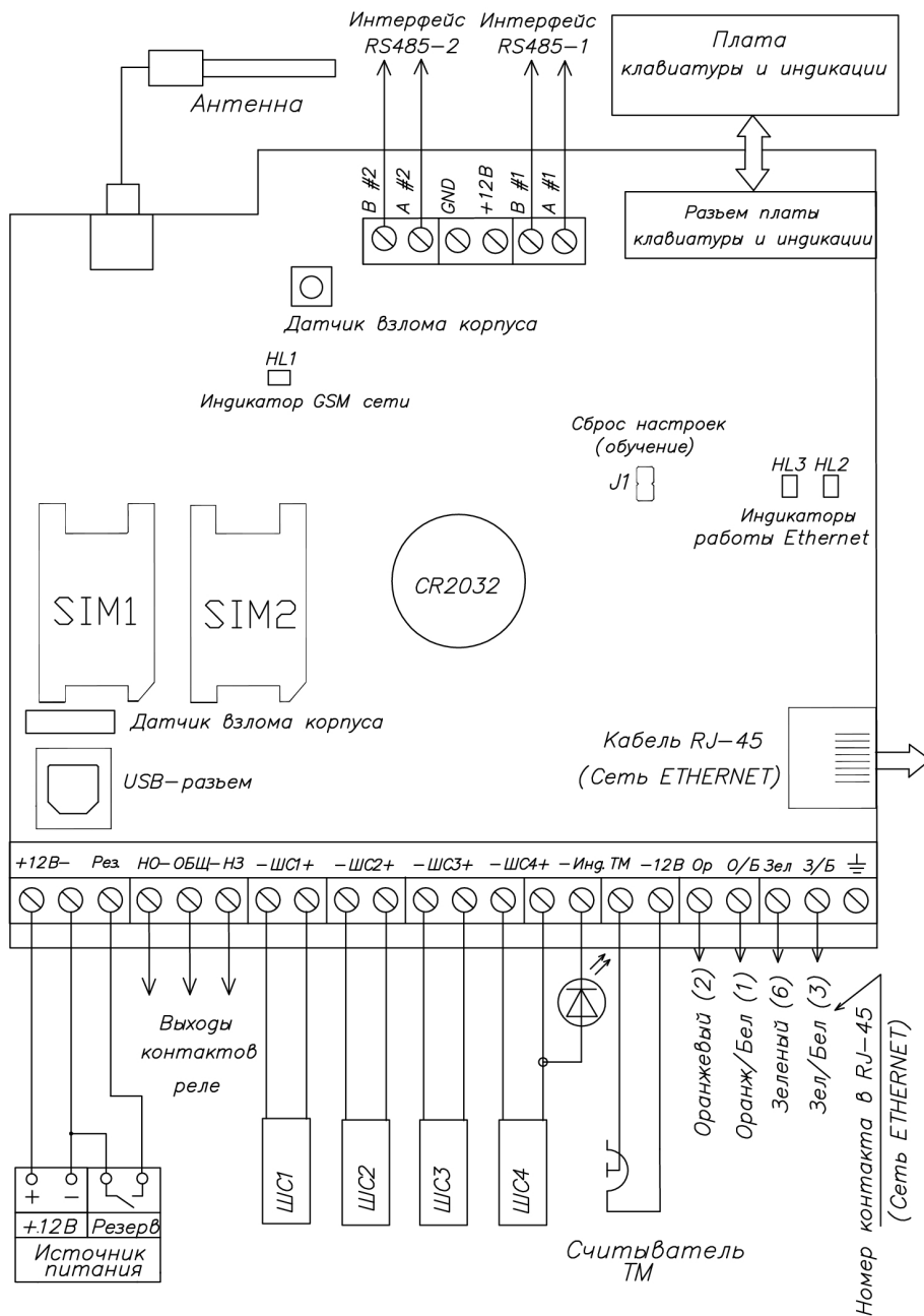
Рисунок 2.6. Назначение разъемов УОО «Юпитер 4 IP/GPRS» (2443, 2463)
