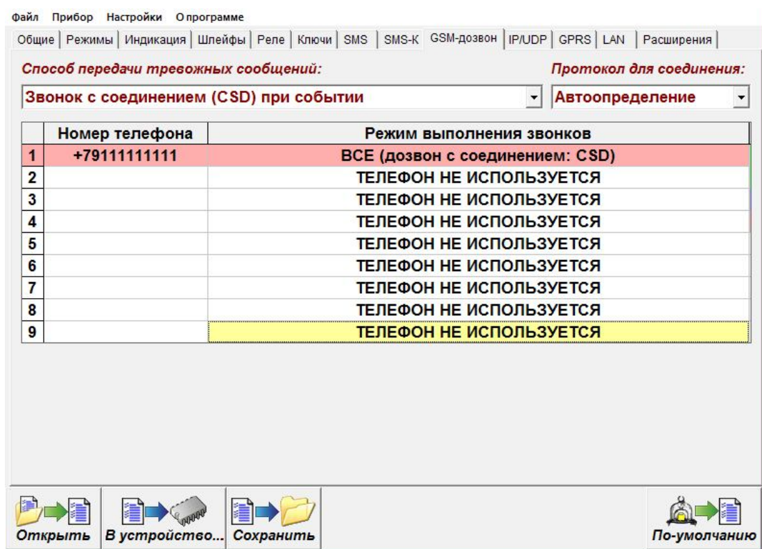
Рисунок 12. Окно программы Конфигуратор, вкладка «GSM-дозвон». Настройка дозвона с соединением
