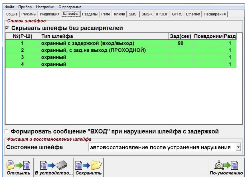
Рисунок 6. Окно программы Конфигуратор, вкладка «Шлейфы» для Юпитер-2445
