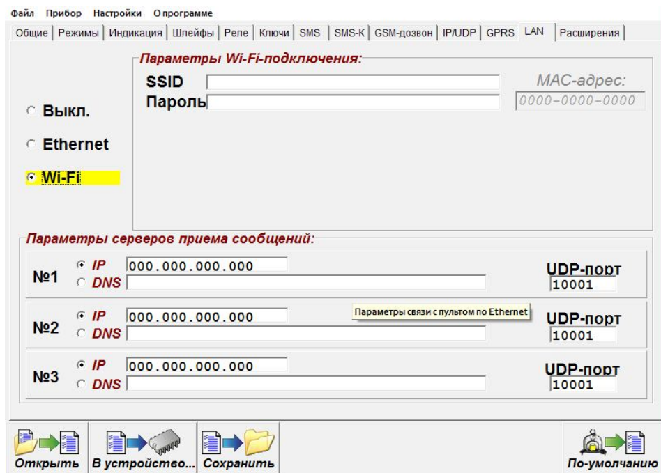
Рисунок 19. Окно программы Конфигуратор, вкладка «LAN»
