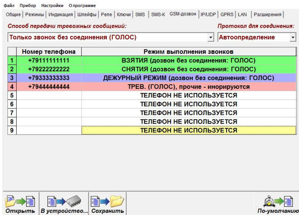
Рисунок 14. Окно программы Конфигуратор, вкладка «GSM-дозвон». Настройка дозвона без соединения
