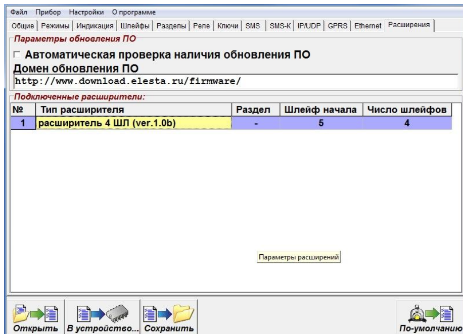
Рисунок 21. Окно программы Конфигуратор, вкладка «Расширения» для прибора Юпитер-2445
