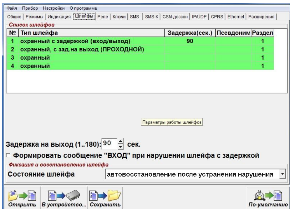
Рисунок 5. Окно программы Конфигуратор, вкладка «Шлейфы» для приборов Юпитер-2413, 2443, 2444, 2463
