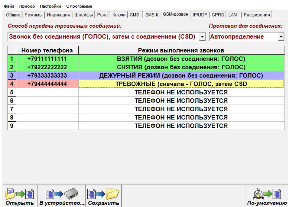
Рисунок 15. Окно программы Конфигуратор, вкладка «GSM-дозвон». Настройка смешанного режима дозвона
