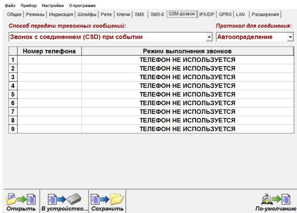
Рисунок 11. Окно программы Конфигуратор, вкладка «GSM-дозвон»
