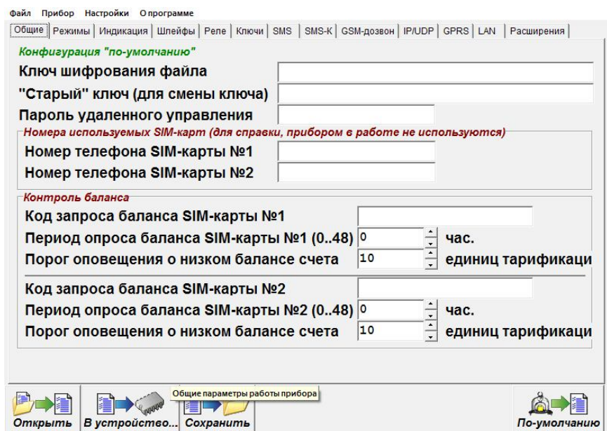
Рисунок 2. Окно программы Конфигуратор, вкладка «Общие»
