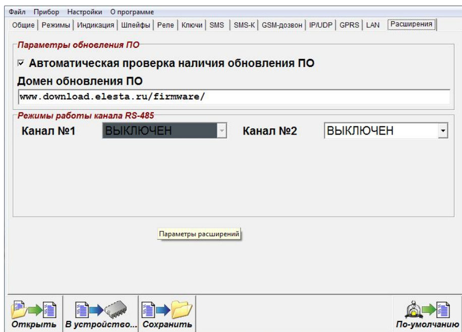
Рисунок 20. Окно программы Конфигуратор, вкладка «Расширения» для приборов Юпитер-2443,2444,2463
