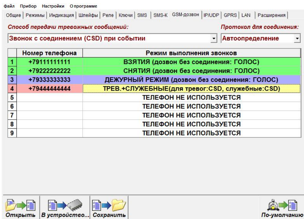
Рисунок 13. Окно программы Конфигуратор, вкладка «GSM-дозвон». Настройка дозвона с соединением для тревожных+служебных сообщений..
