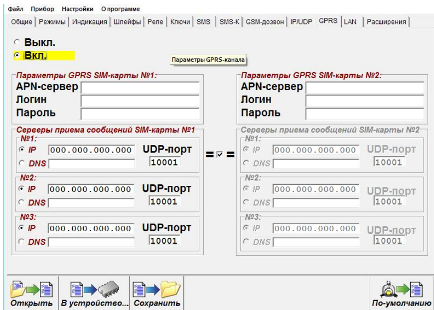
Рисунок 17. Окно программы Конфигуратор, вкладка «GPRS»
