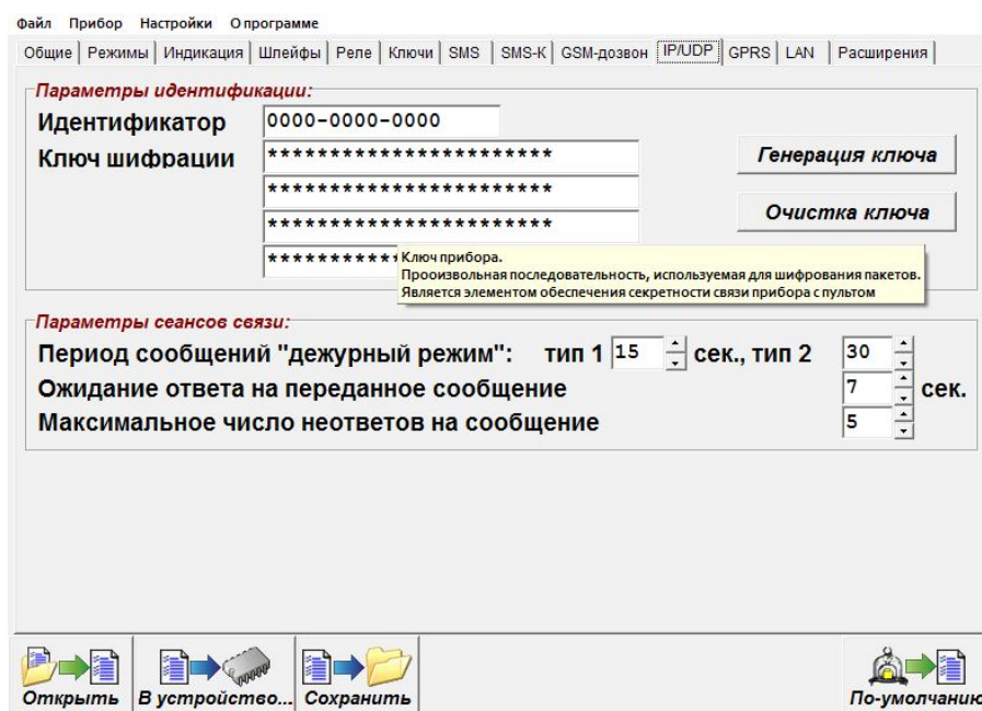
Рисунок 15. Окно программы Конфигуратор, вкладка «IP/UDP»
