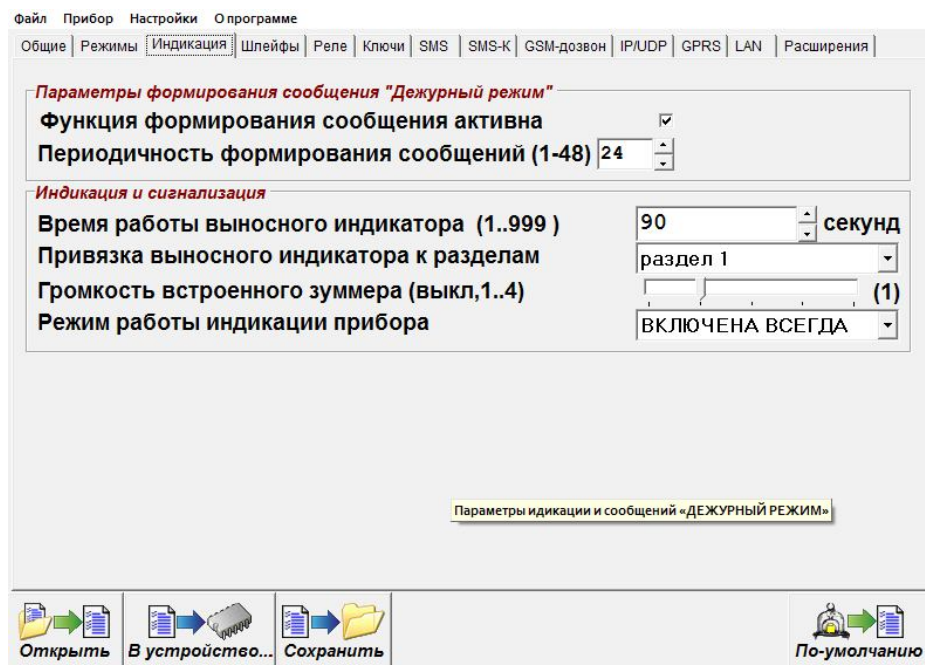
Рисунок 4. Окно программы Конфигуратор, вкладка «Индикация»
