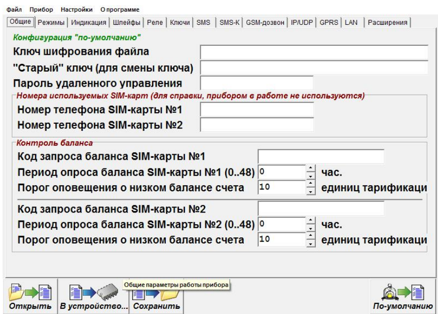
Рисунок 2. Окно программы Конфигуратор, вкладка «Общие»
