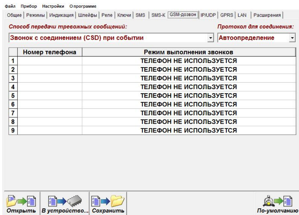
Рисунок 10. Окно программы Конфигуратор, вкладка «GSM-дозвон»
