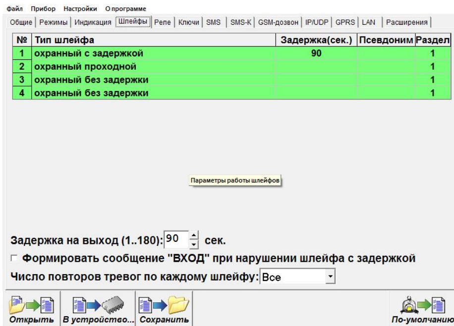
Рисунок 5. Окно программы Конфигуратор, вкладка «Шлейфы»
