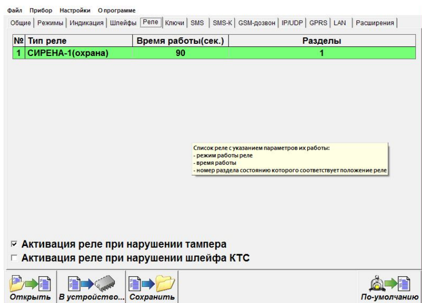
Рисунок 6. Окно программы Конфигуратор, вкладка «Реле»
