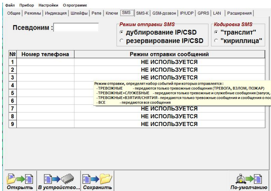
Рисунок 8. Окно программы Конфигуратор, вкладка «SMS»
