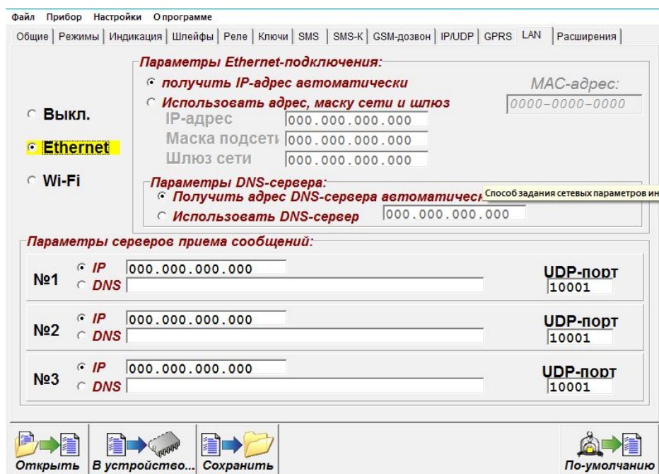
Рисунок 17. Окно программы Конфигуратор, вкладка «LAN»
