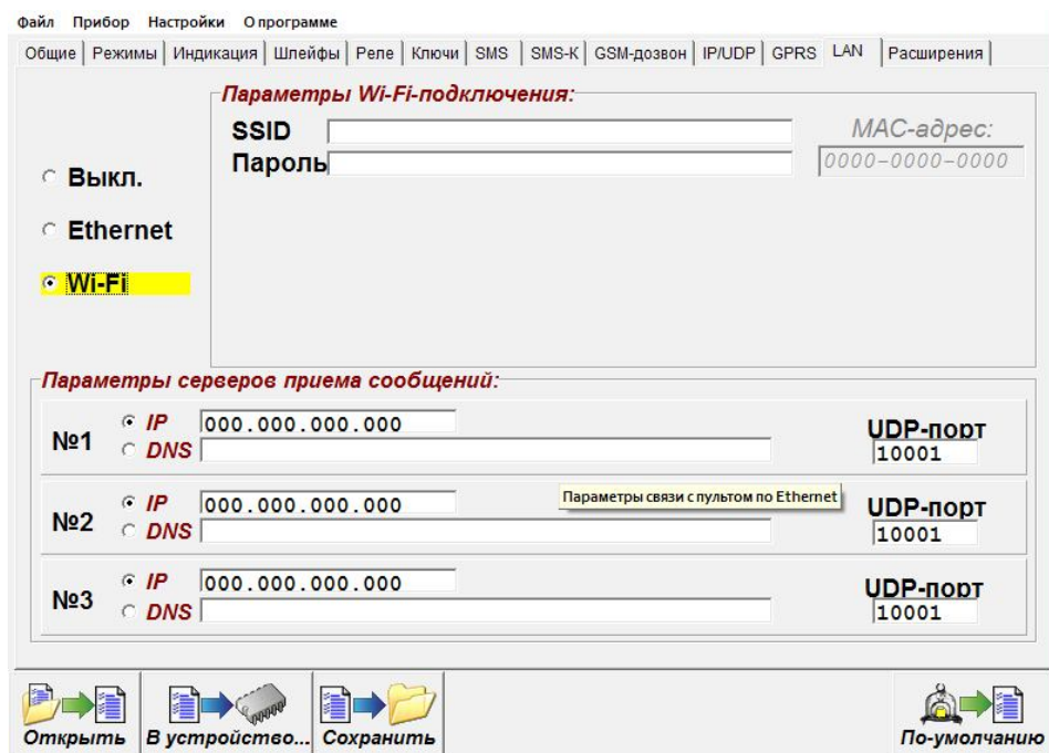
Рисунок 18. Окно программы Конфигуратор, вкладка «LAN»
