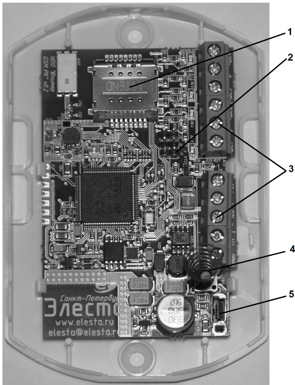
Рисунок 2.2 - Вид прибора с открытой крышкой. Плата версии 0.2 (Юпитер-2420)
