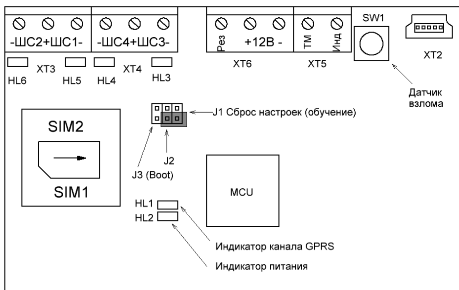
Рисунок 3.2 - Плата версии 0.2. Взаимное замыкание переключек
