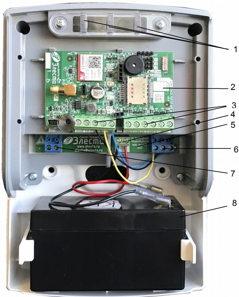
Рисунок 2.7 - Прибор Юпитер-2428 с открытой крышкой
