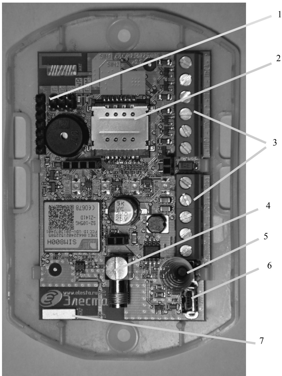
Рисунок 2.3 - Вид прибора с открытой крышкой. Плата версии 0.6 (Юпитер-2426)
