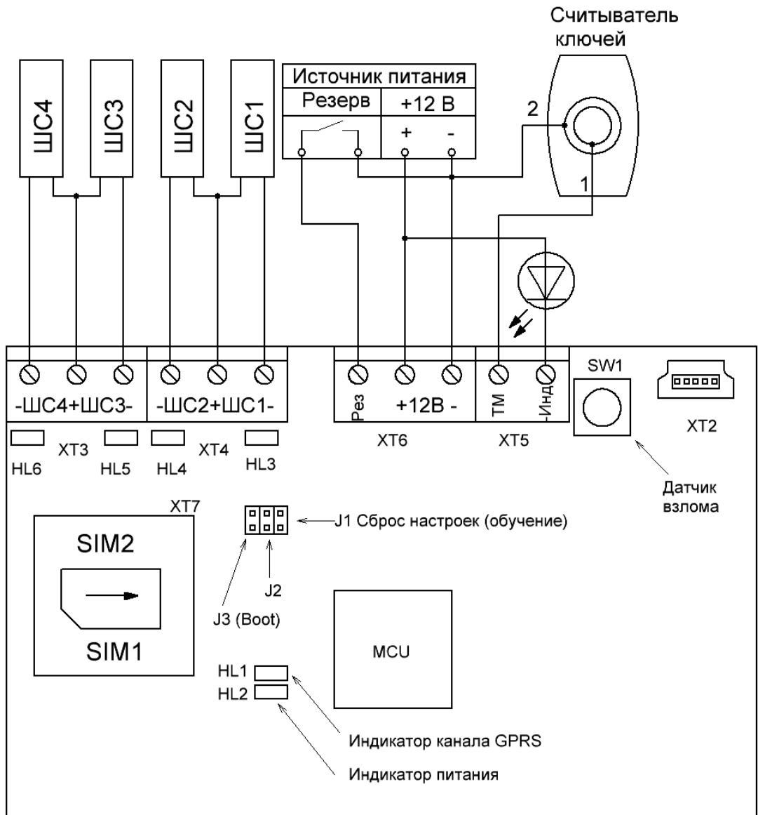
Рисунок 2.5 - Подключение внешних элементов прибора (плата версии 0.2)
