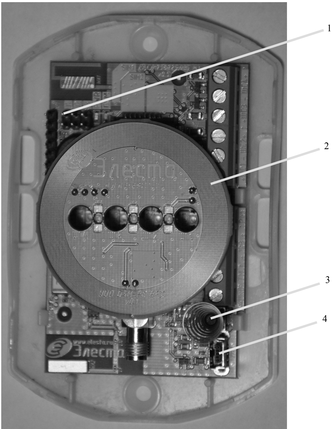
Рисунок 2.4 - Вид прибора с открытой крышкой. Плата версии 0.6 (Юпитер-2427)
