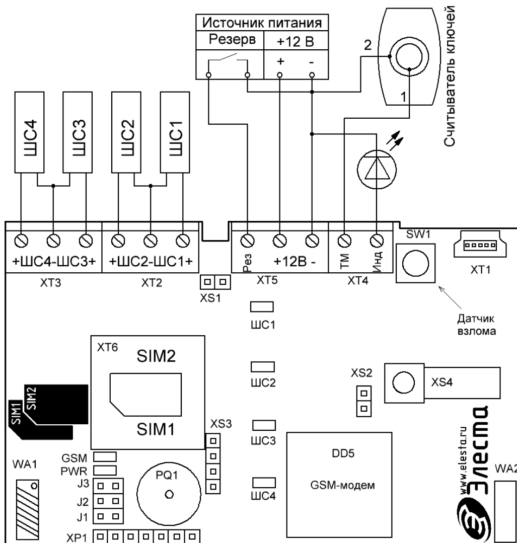
Рисунок 2.8 - Назначение разъемов прибора
