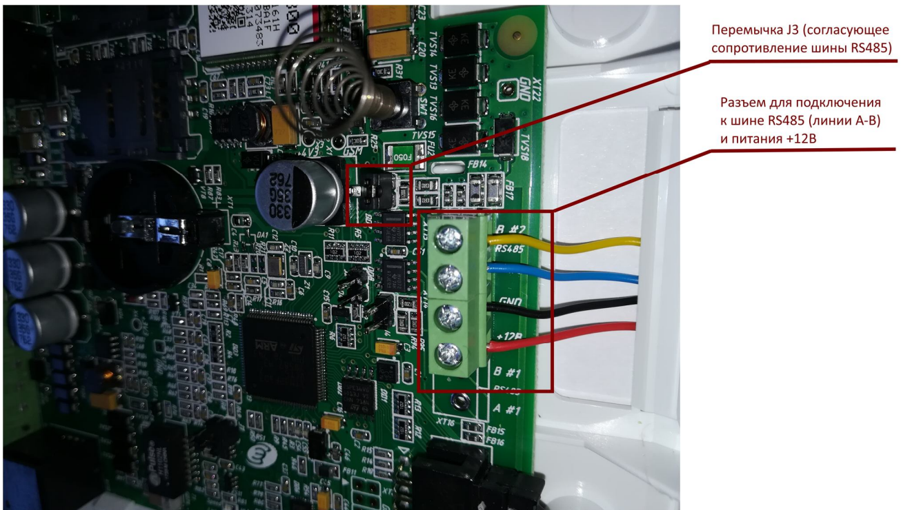
Рисунок 2. Подключение УОО к линии RS485.
