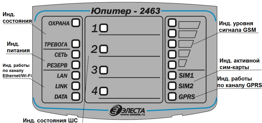
Рисунок 3. Внешний вид панели индикации
